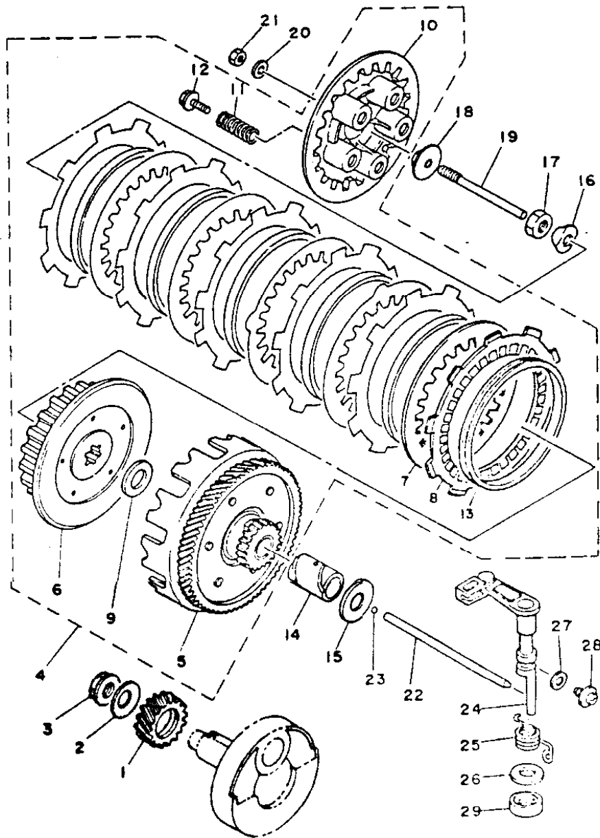
FIG. 05 - FRICÇÃO
