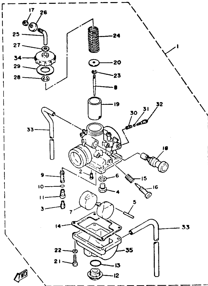
FIG. 12 - CARBURADOR
