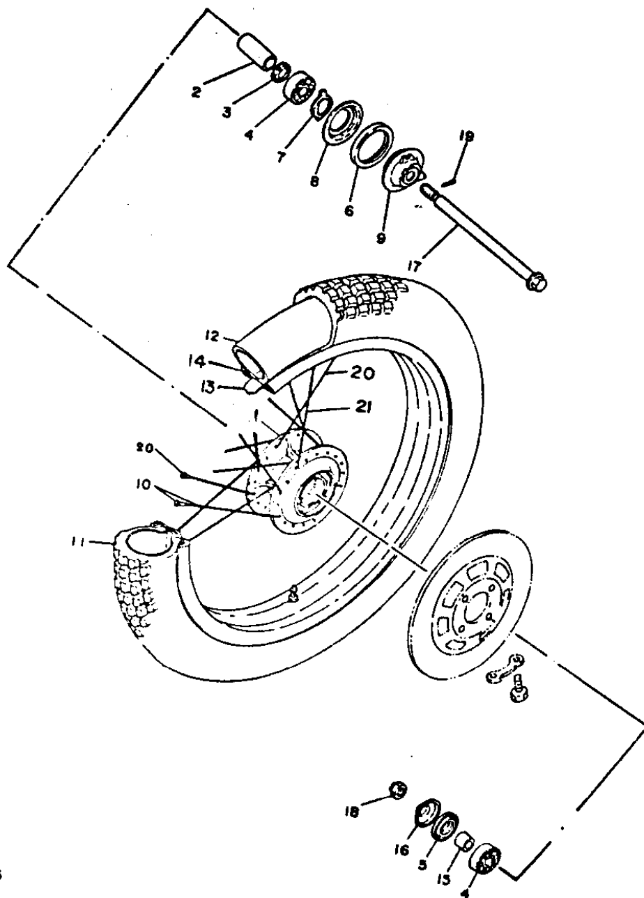
FIG. 28 - RODA DIANTEIRA
