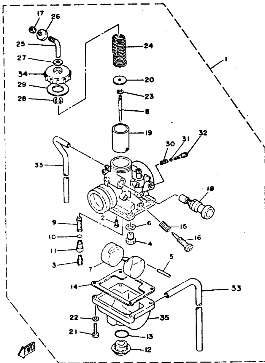
FIG. 12 - CARBURADOR
