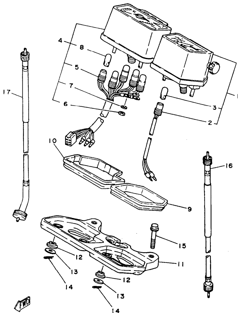
FIG. 39 - VELOCÍMETRO E TACOMETRO
