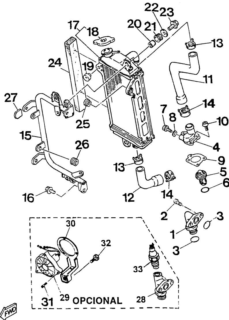
FIG. 04 - RADIADOR
