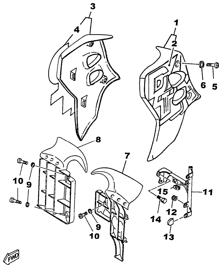
FIG. 19 - TOMADA DE AR - PAINÉIS SUPORTE DO PAINEL
