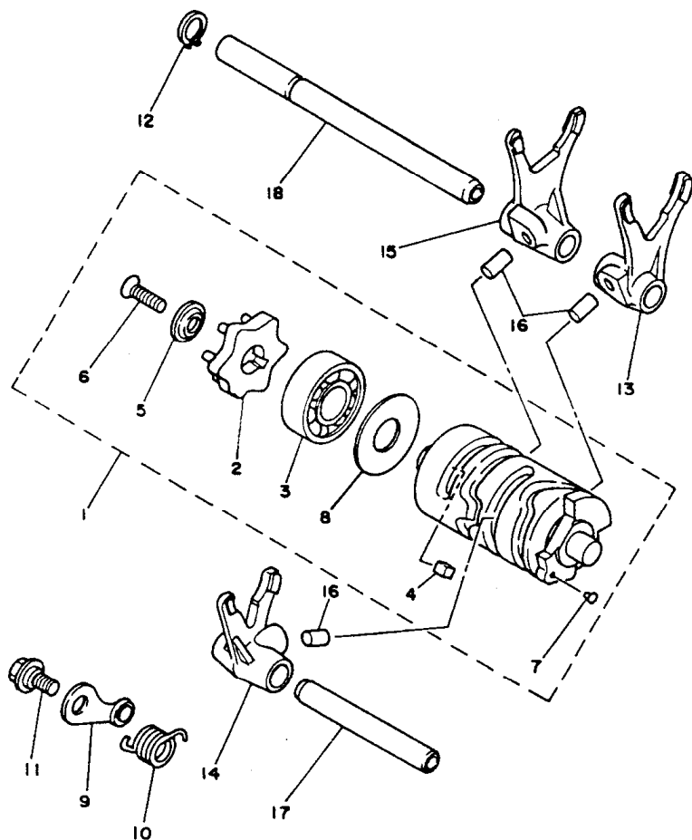
FIG. 15 - EIXO TRAMBULADOR
