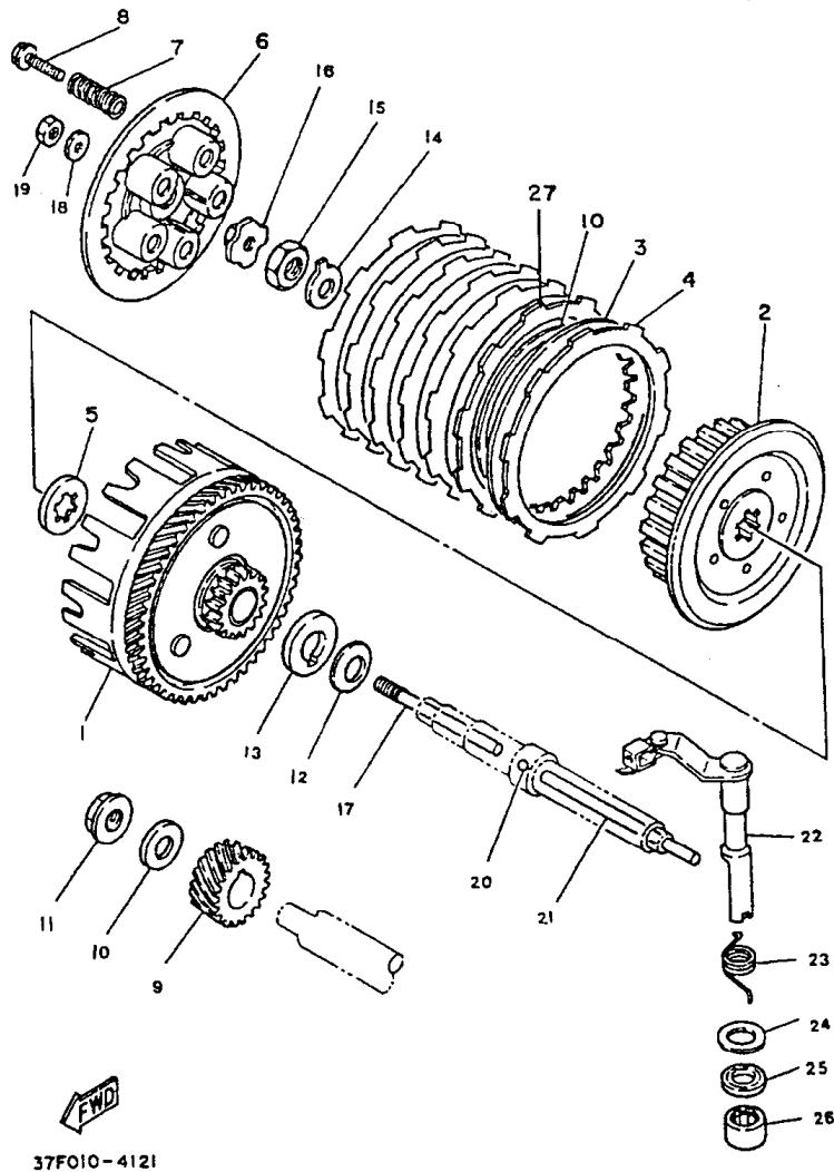
FIG. 12 - FRICÇÃO
