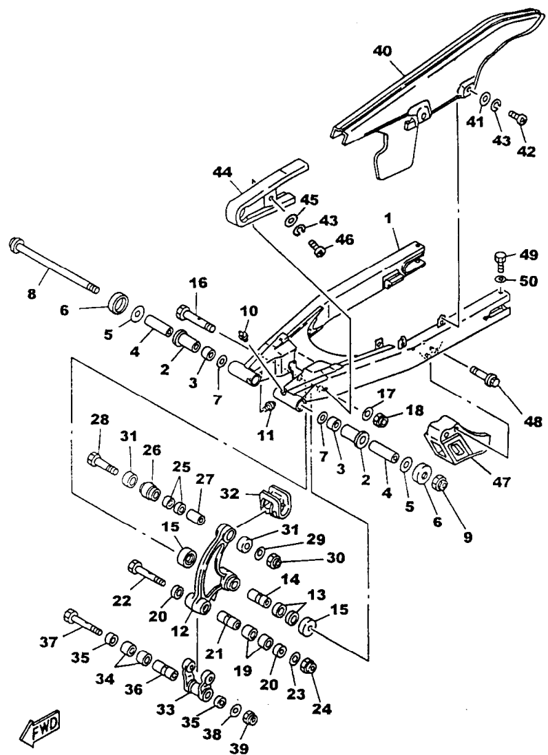
FIG. 22 - GARFO TRASEIRO
