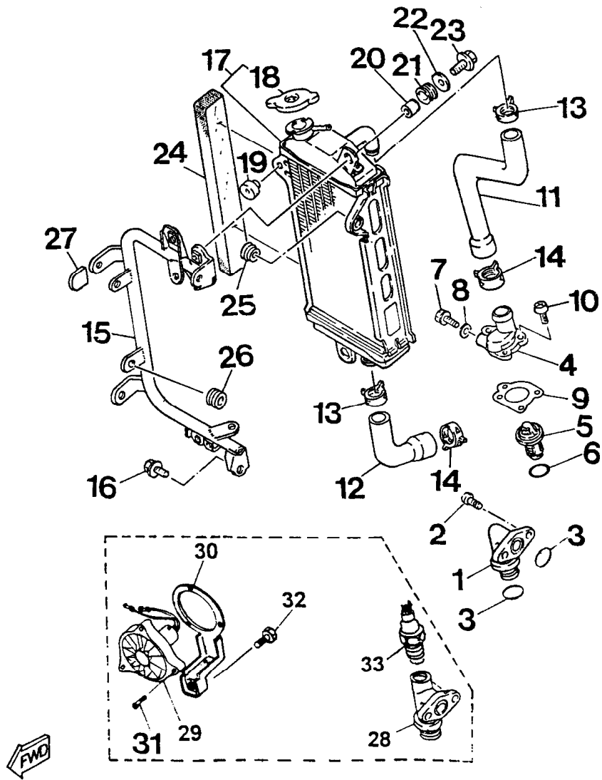
FIG. 04 - RADIADOR
