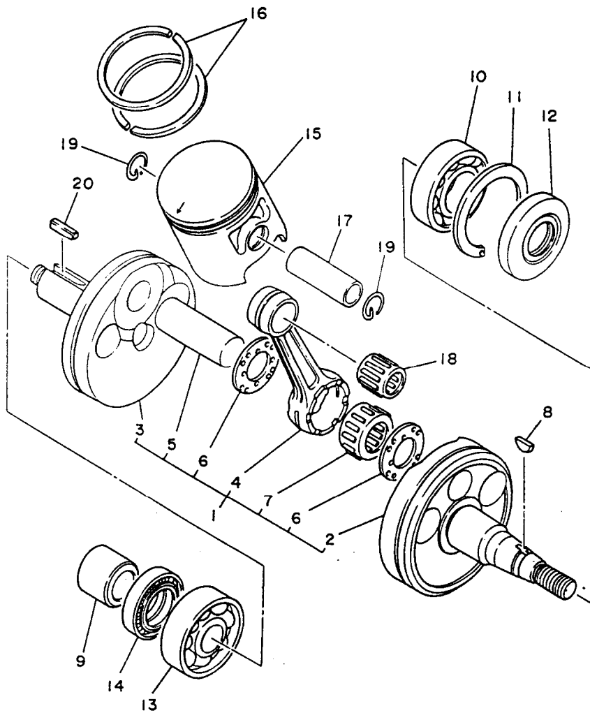
FIG. 2 - VIRABREQUIM E PISTÃO
