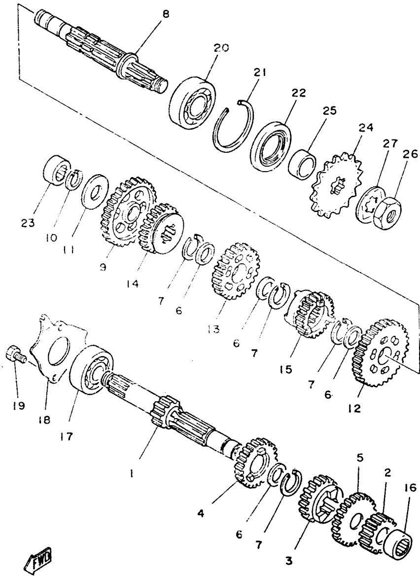
FIG. 11 - TRANSMISSÃO
