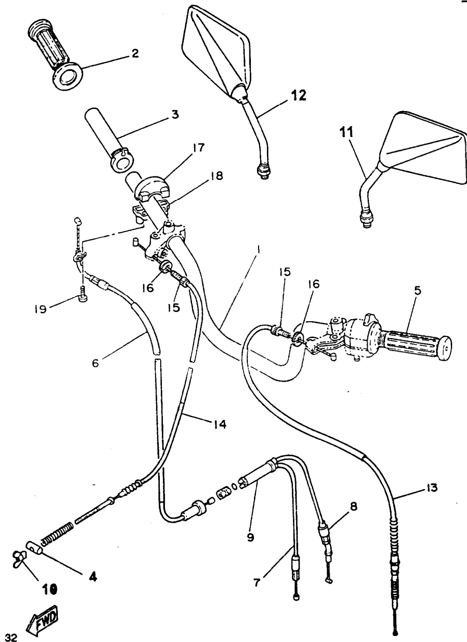
FIG. 26 - GUIDÃO E CABOS
