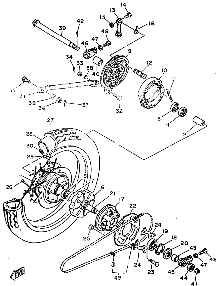
FIG. 25 - RODA TRASEIRA
