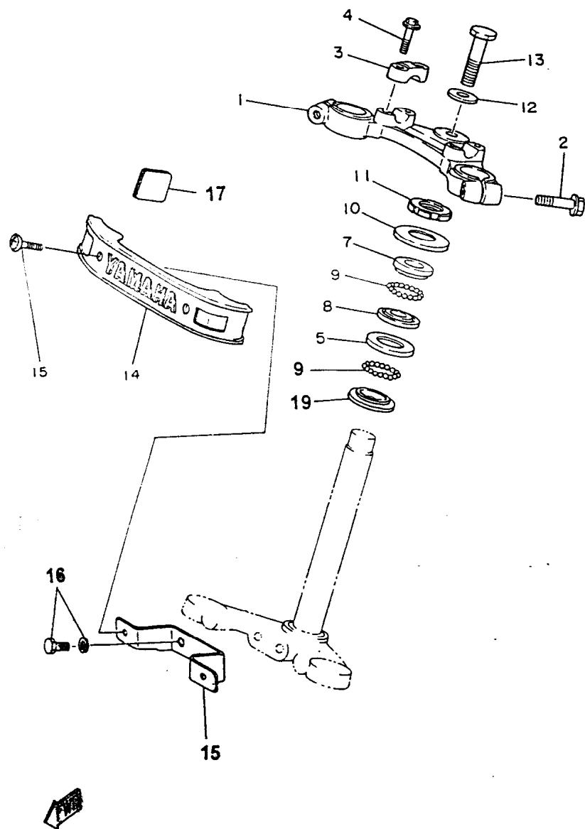
FIG. 20 - MESA DO GUIDÃO
