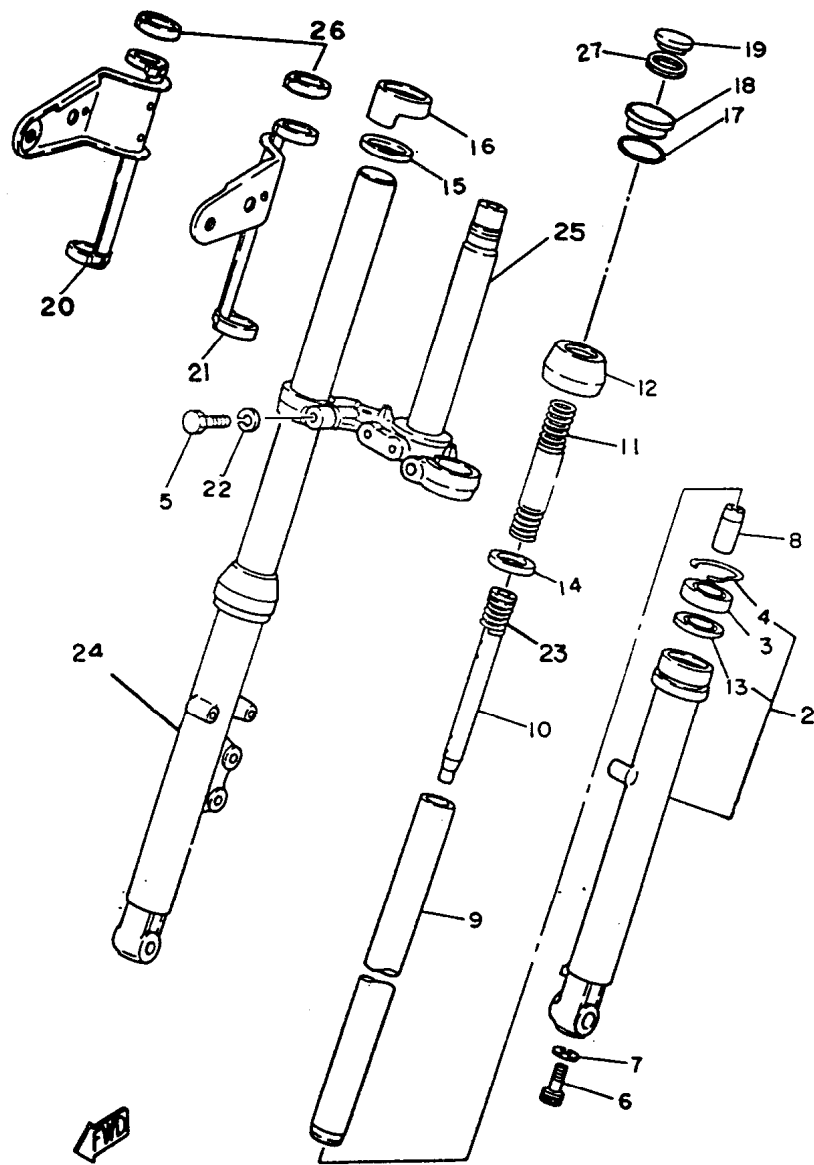
FIG. 21 - GARFO TELESCÓPICO
