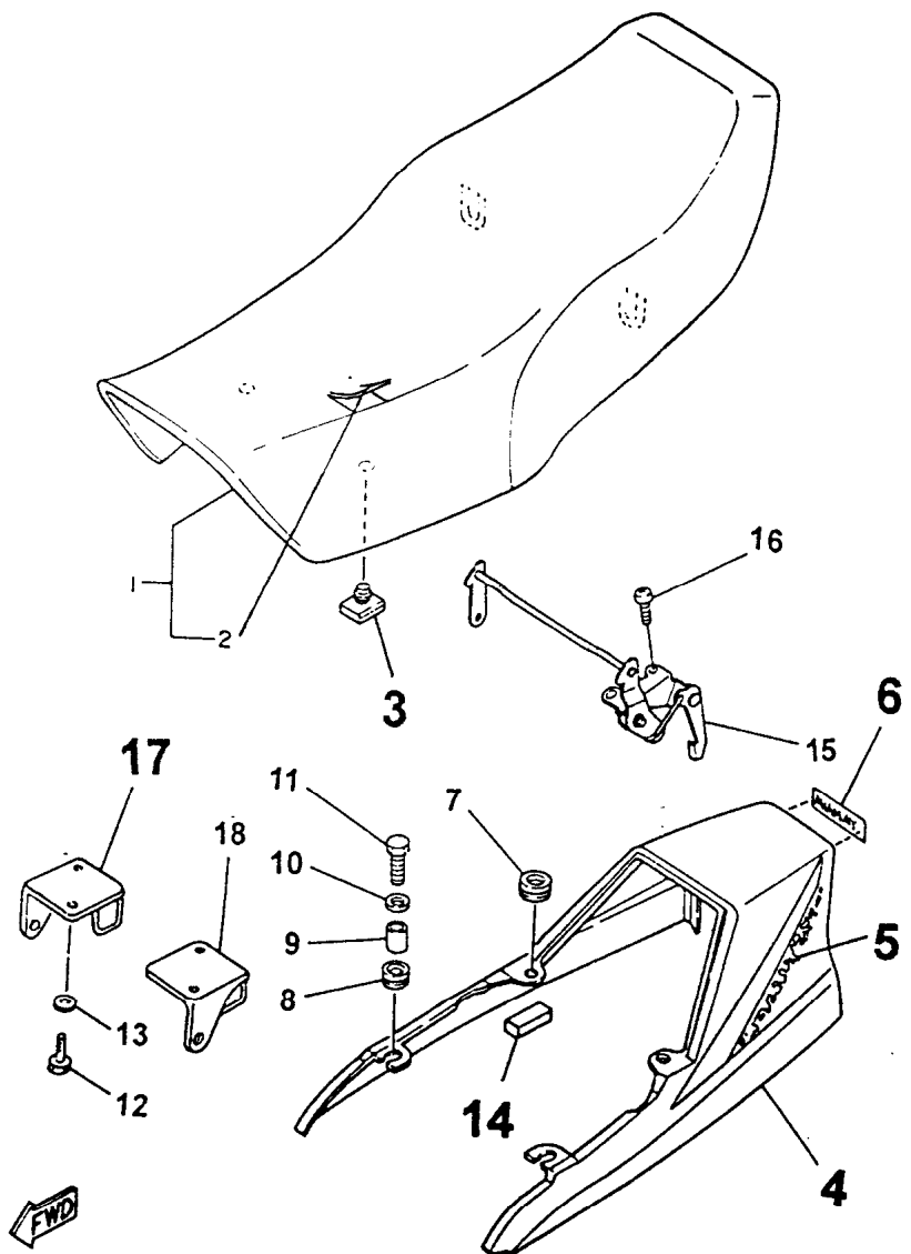
FIG. 23 - ASSENTO E RABETA
