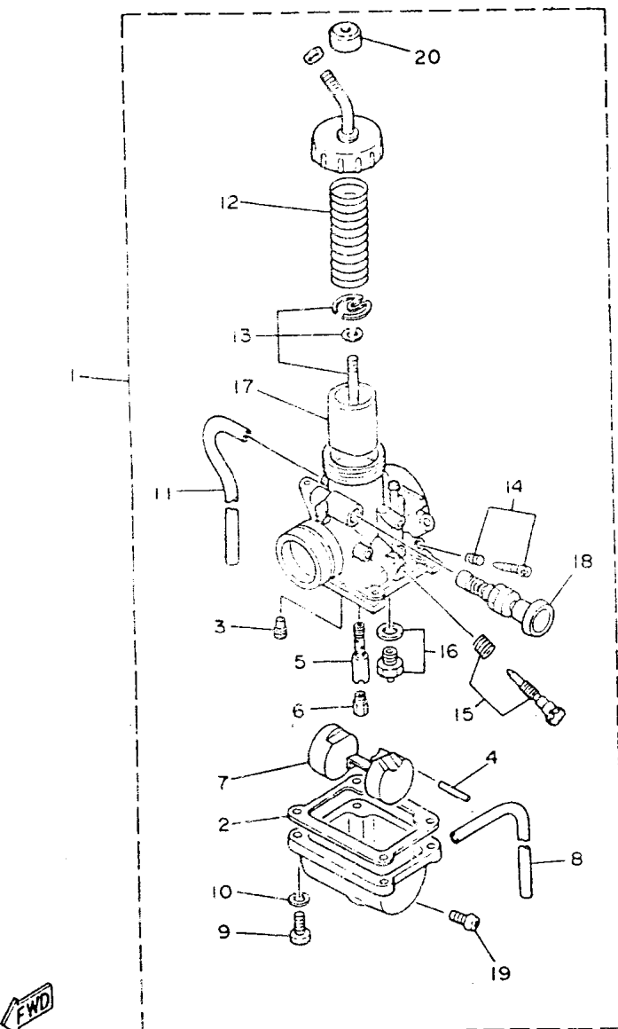
FIG. 5 - CARBURADOR
