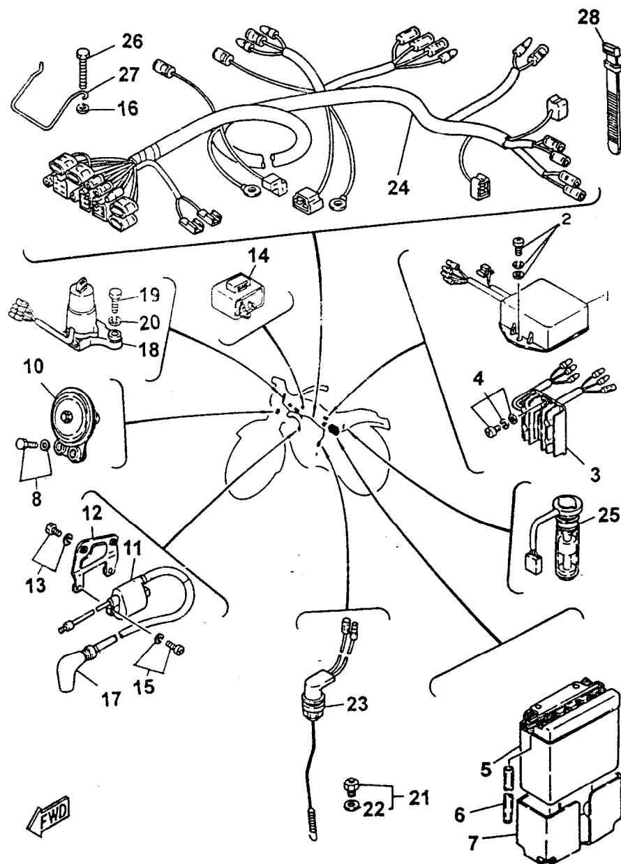
FIG. 33 - SISTEMA ELÉTRICO
