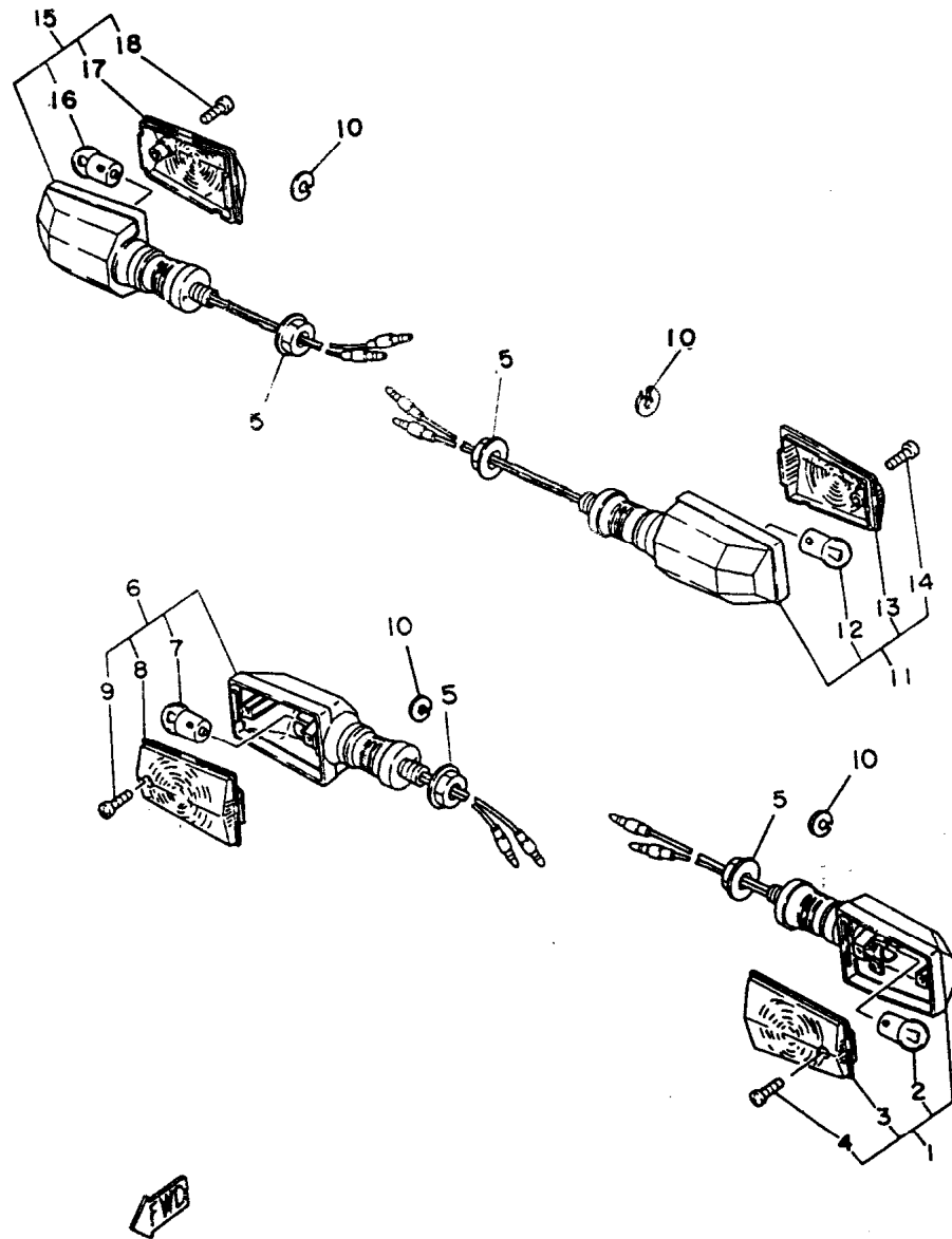
FIG. 29 - SINALIZADORES (PISCA-PISCA)
