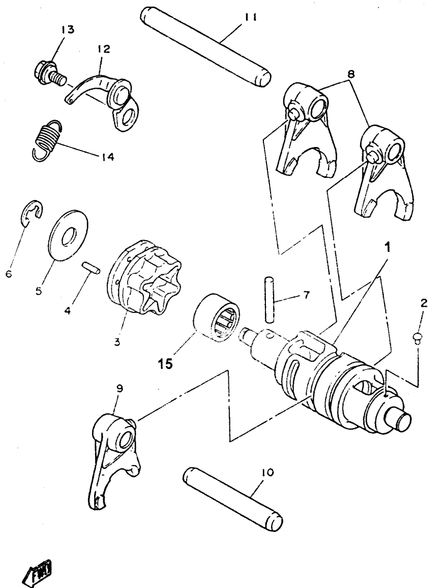
FIG. 13 - EIXO TRAMBULADOR
