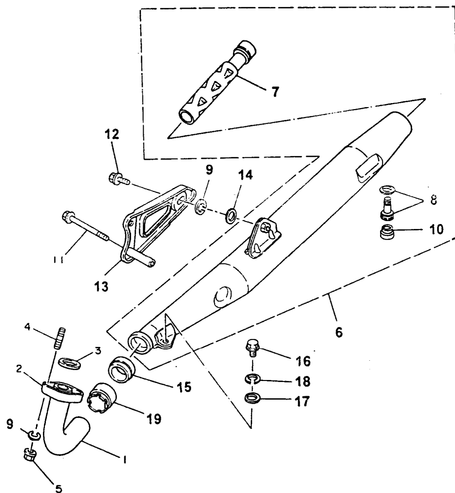
FIG. 06 - ESCAPAMENTO
