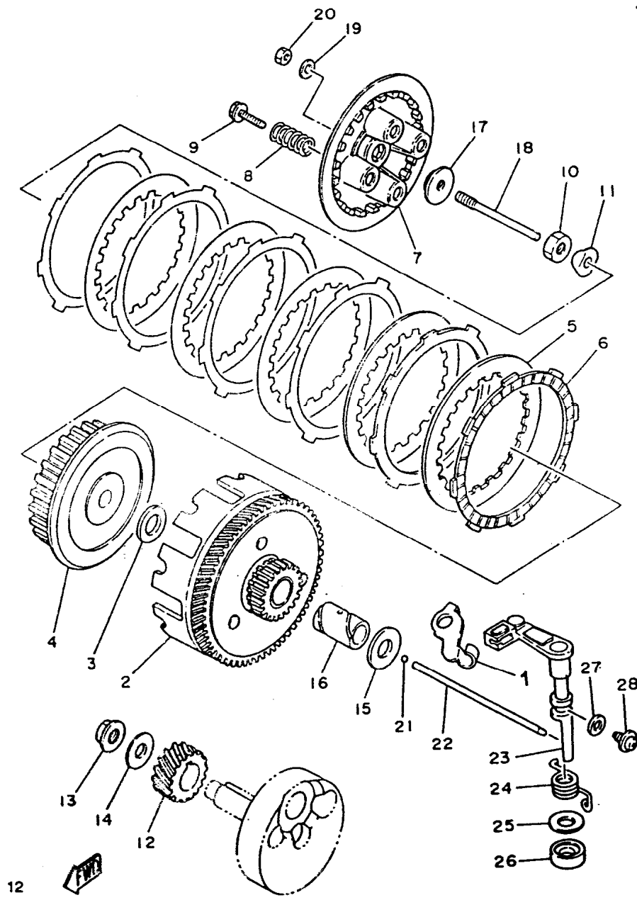
FIG. 10 - FRICÇÃO
