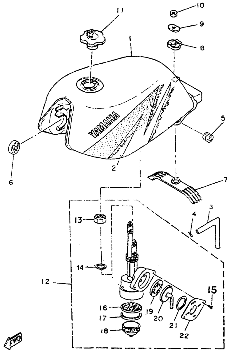
FIG. 22 - TANQUE DE GASOLINA
