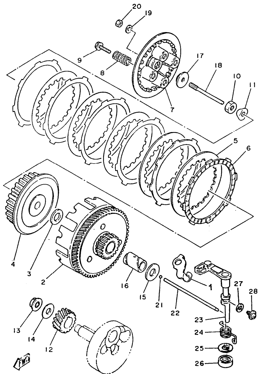
FIG. 10 - FRICÇÃO
