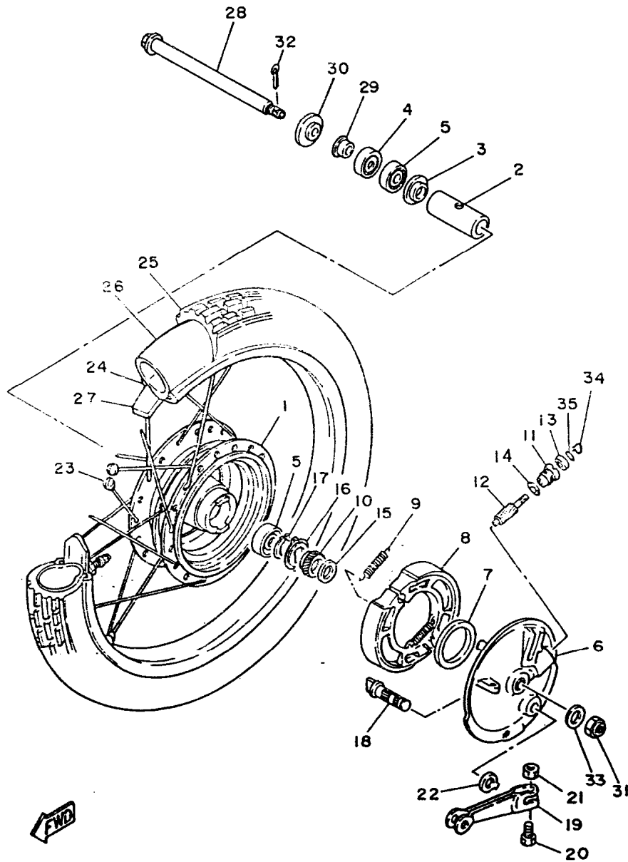
FIG. 24 - RODA DIANTEIRA
