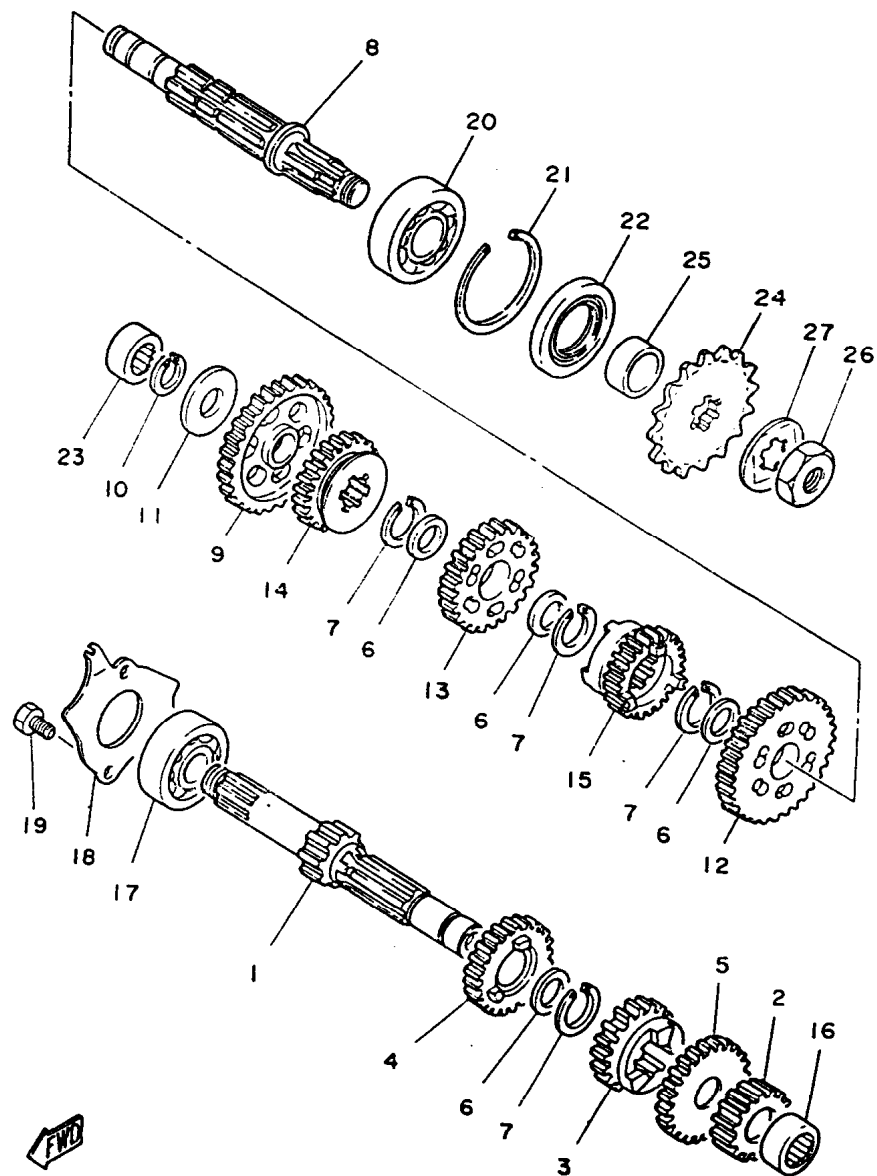
FIG. 11 - TRANSMISSÃO
