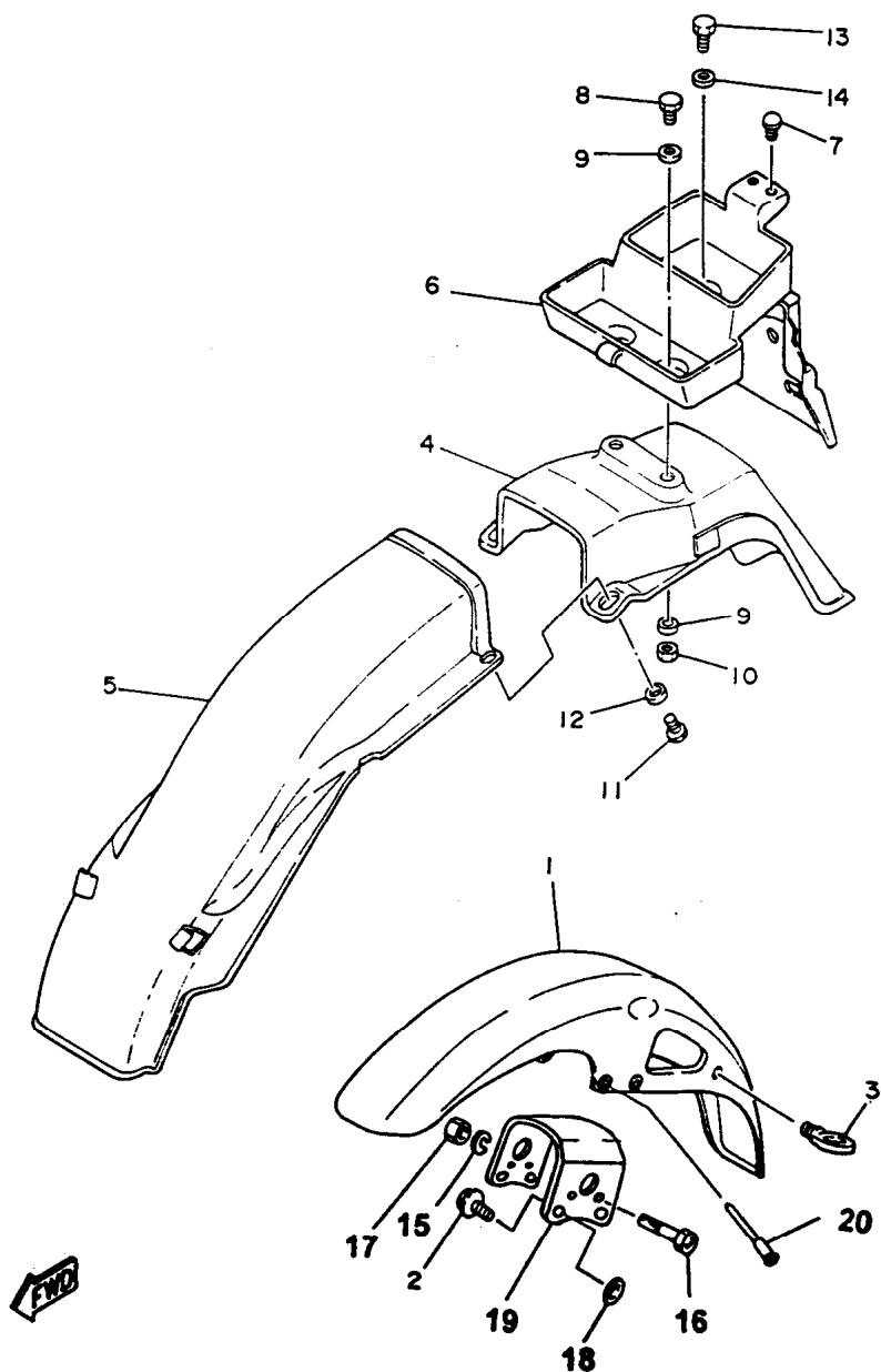
FIG. 16 - PÁRA-LAMA DIANTEIRO E TRASEIRO
