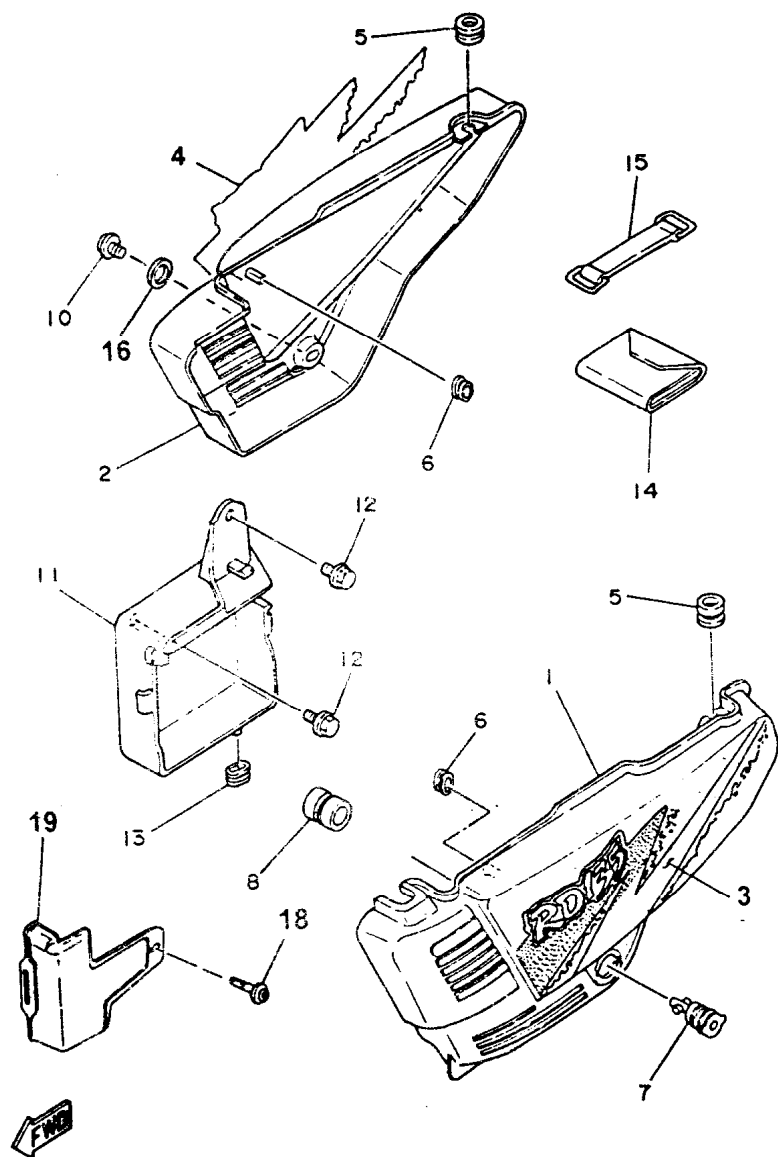
FIG. 17 - TAMPAS LATERAIS
