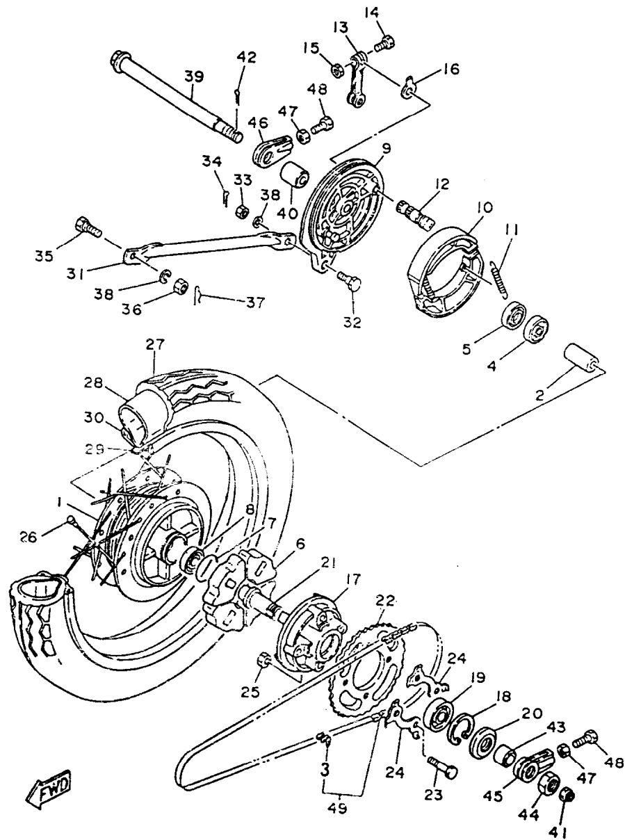
FIG. 25 - RODA TRASEIRA
