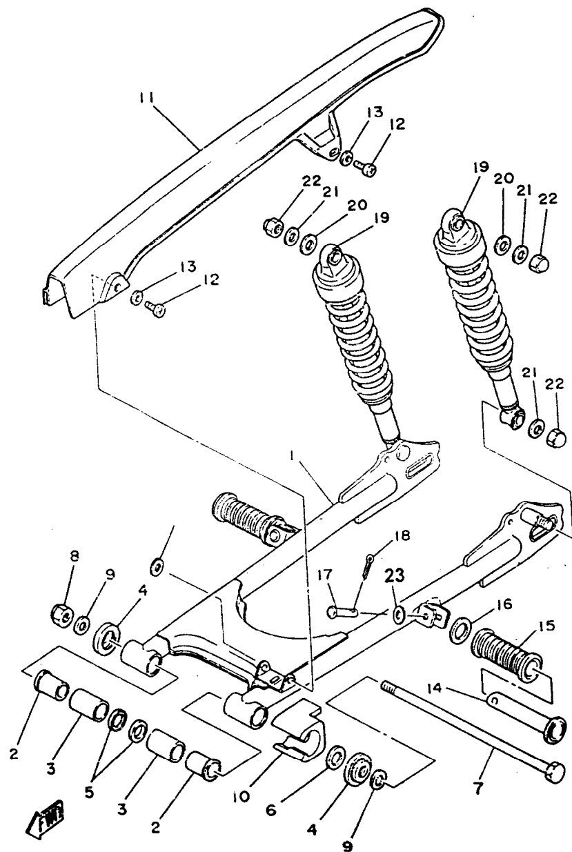
FIG. 19 - GARFO TRASEIRO
