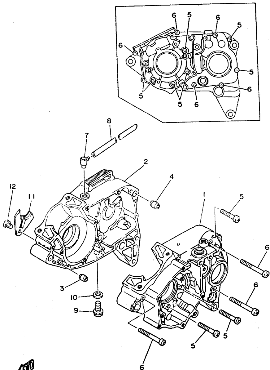
FIG. 07 - CARÇAÇA DO MOTOR
