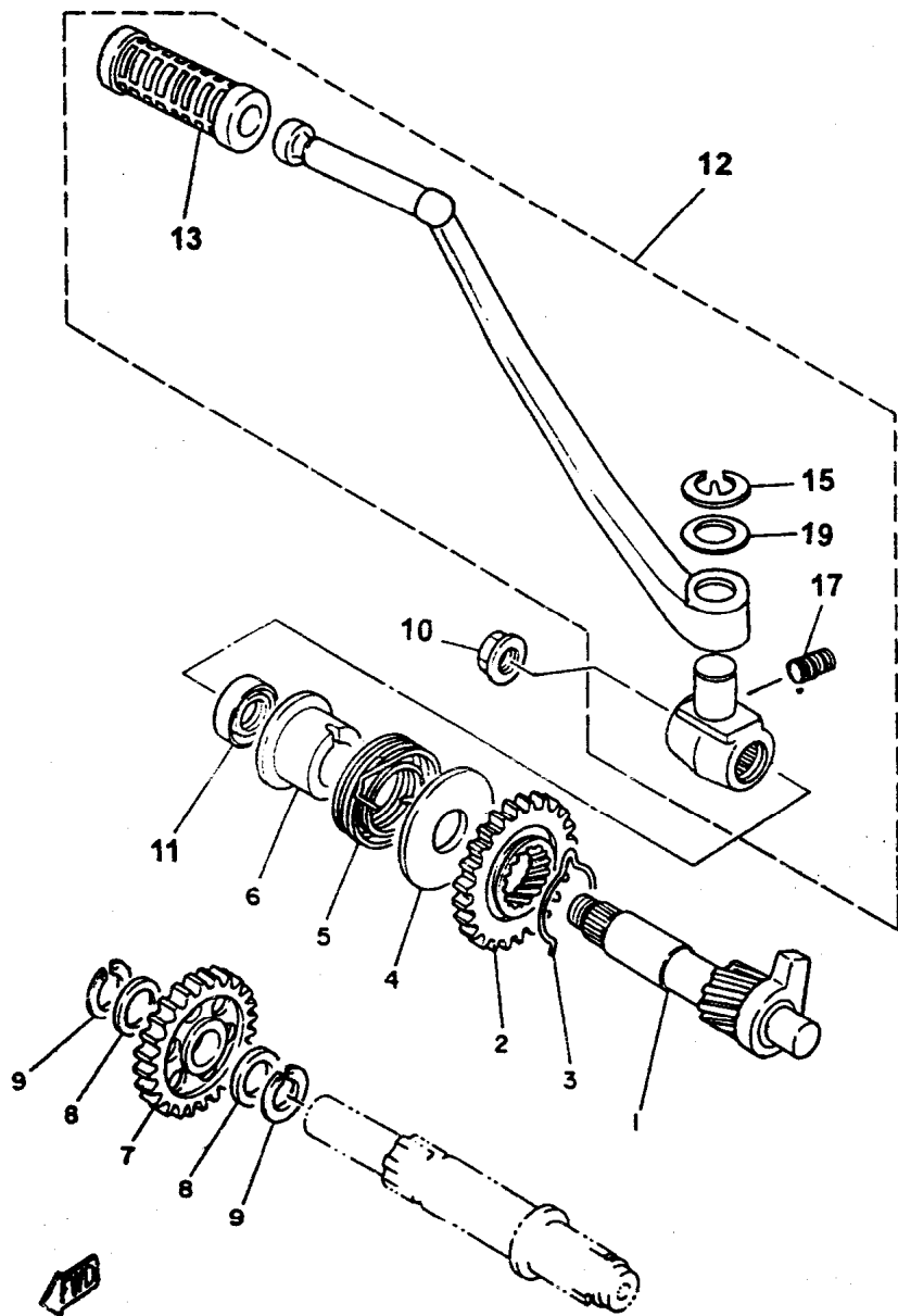
FIG. 9 - EIXO DO PEDAL DE PARTIDA
