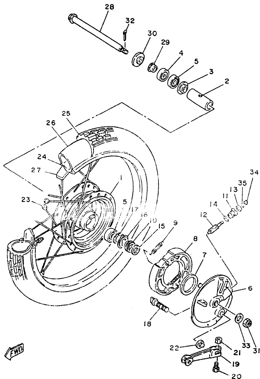
FIG. 24 - RODA DIANTEIRA
