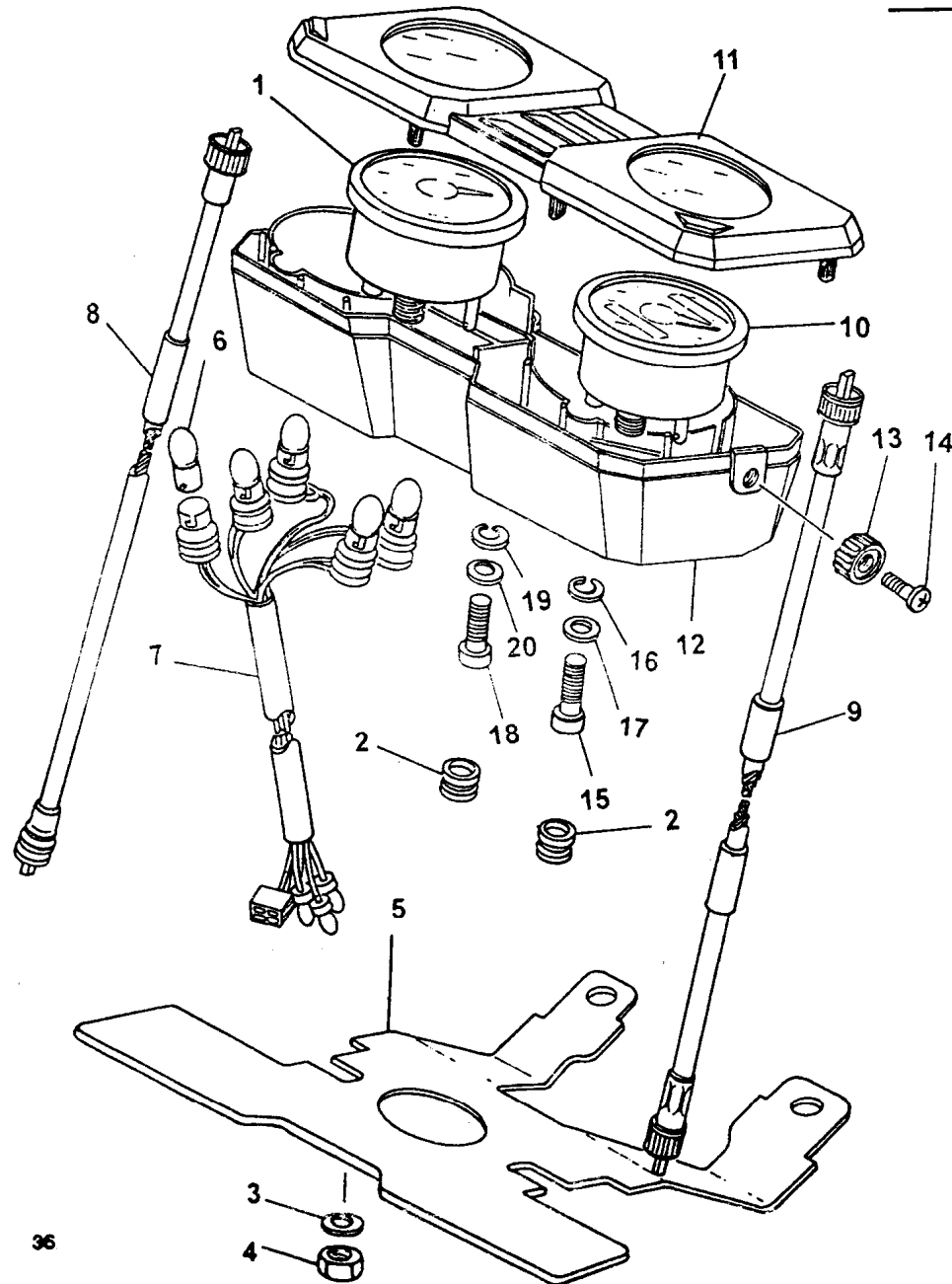
FIG. 30 - PAINEL DE INSTRUMENTOS
