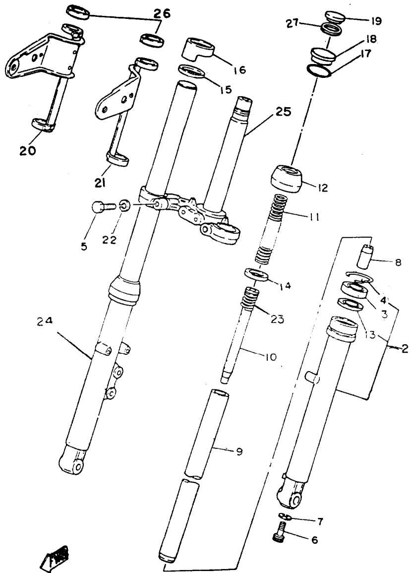
FIG. 21 - GARFO TELESCÓPICO
