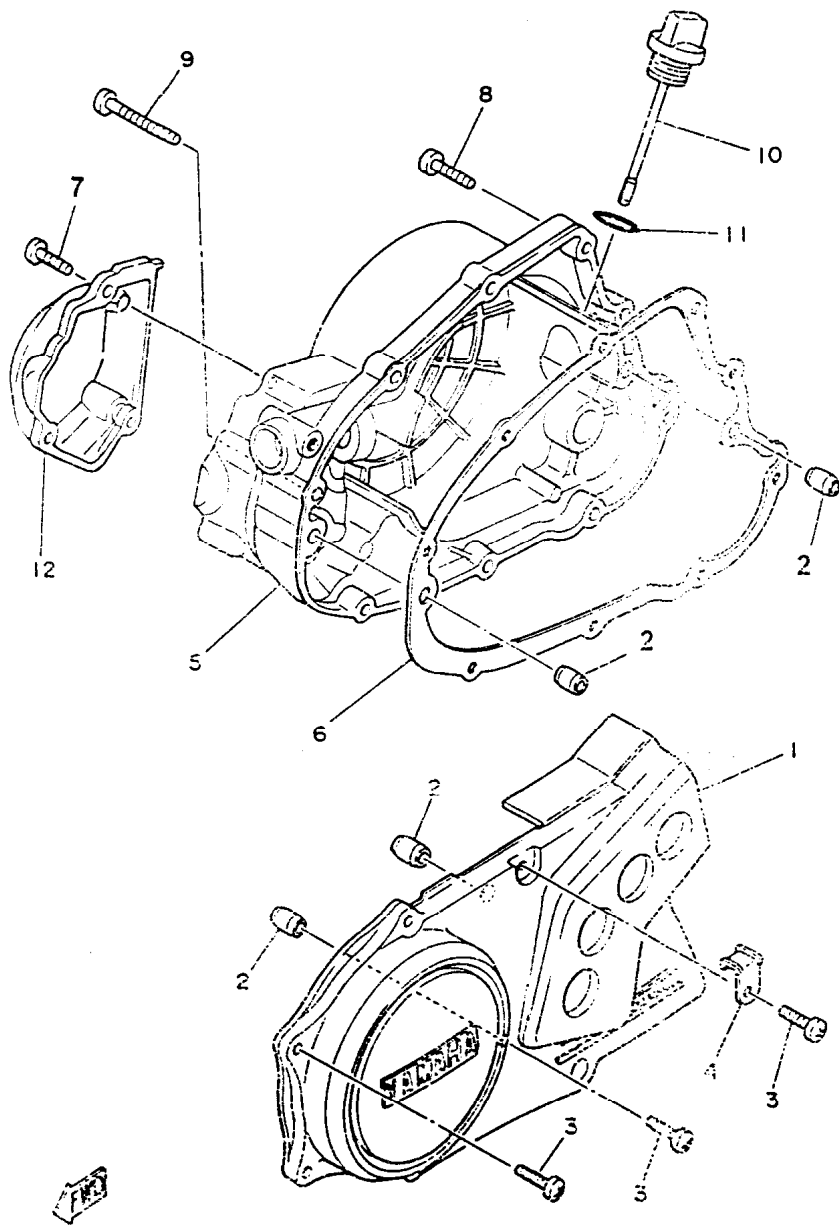
FIG. 8 - TAMPA DA CARÇAÇA
