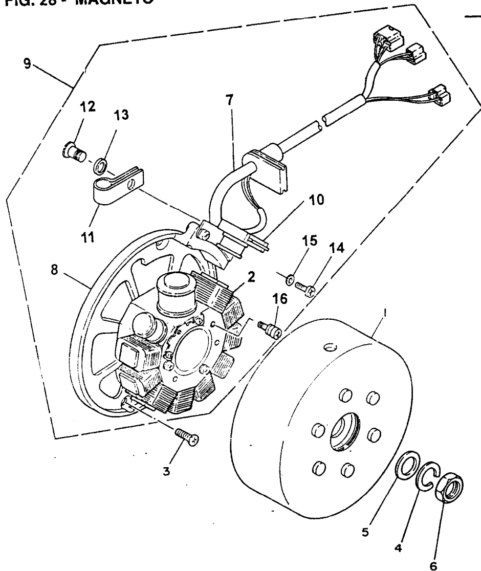
FIG. 28 - MAGNETO
