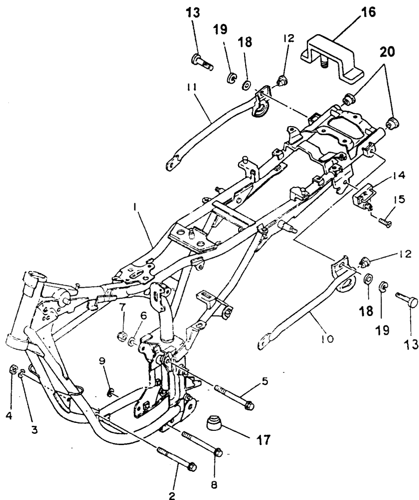
FIG. 15 - CHASSI
