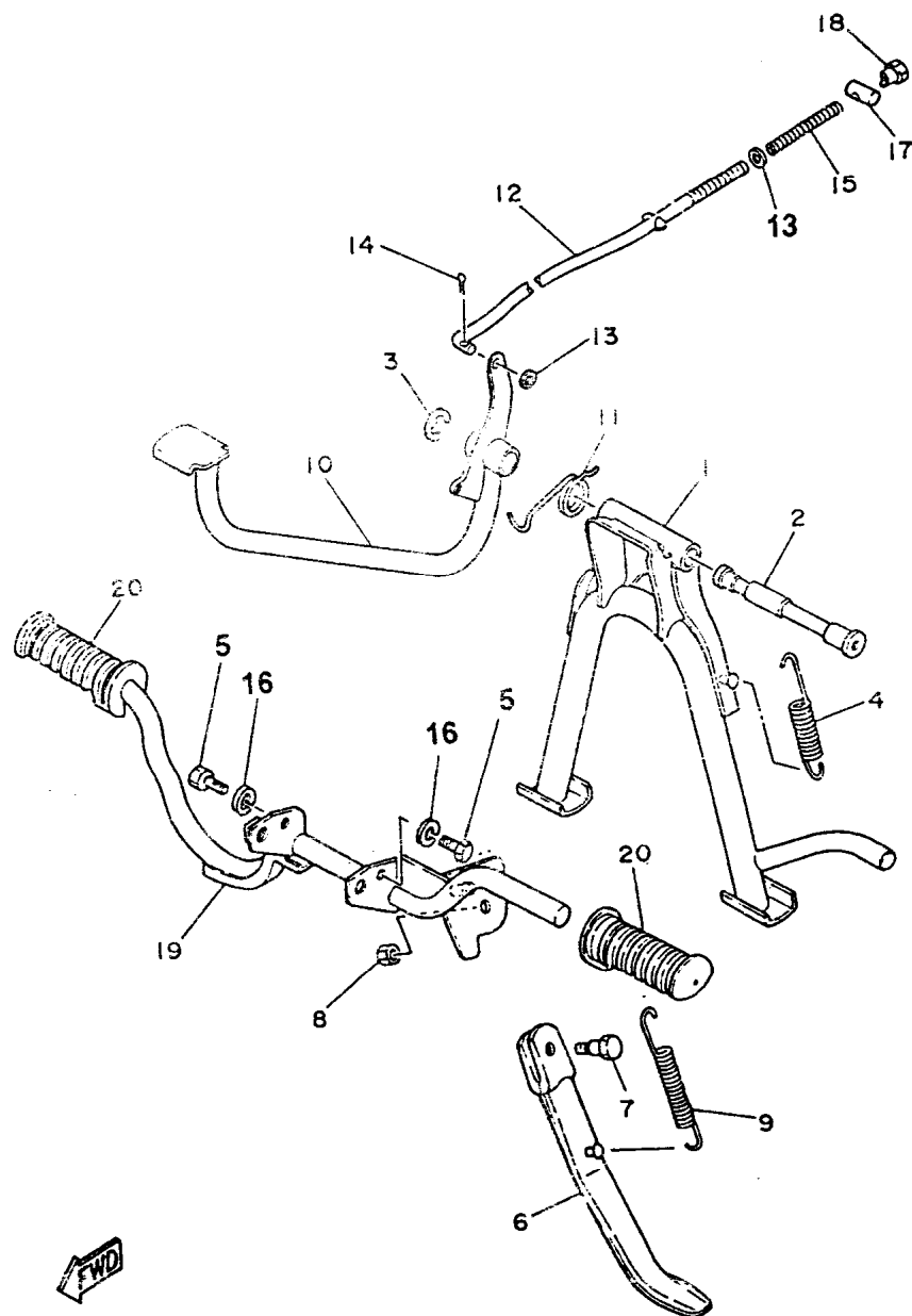
FIG. 27 - CAVALETE - ESTRIBOS PEDAL DE FREIO
