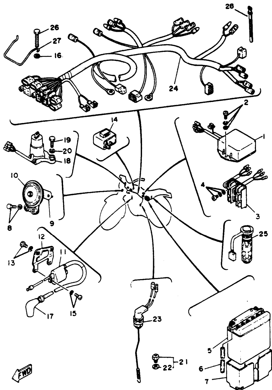
FIG. 33 – SISTEMA ELÉTRICO
