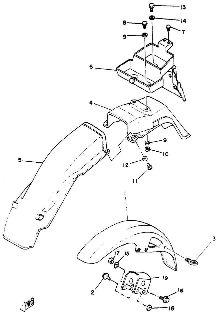
FIG. 16 – PARALAMA DIANTEIRO E TRASEIRO
