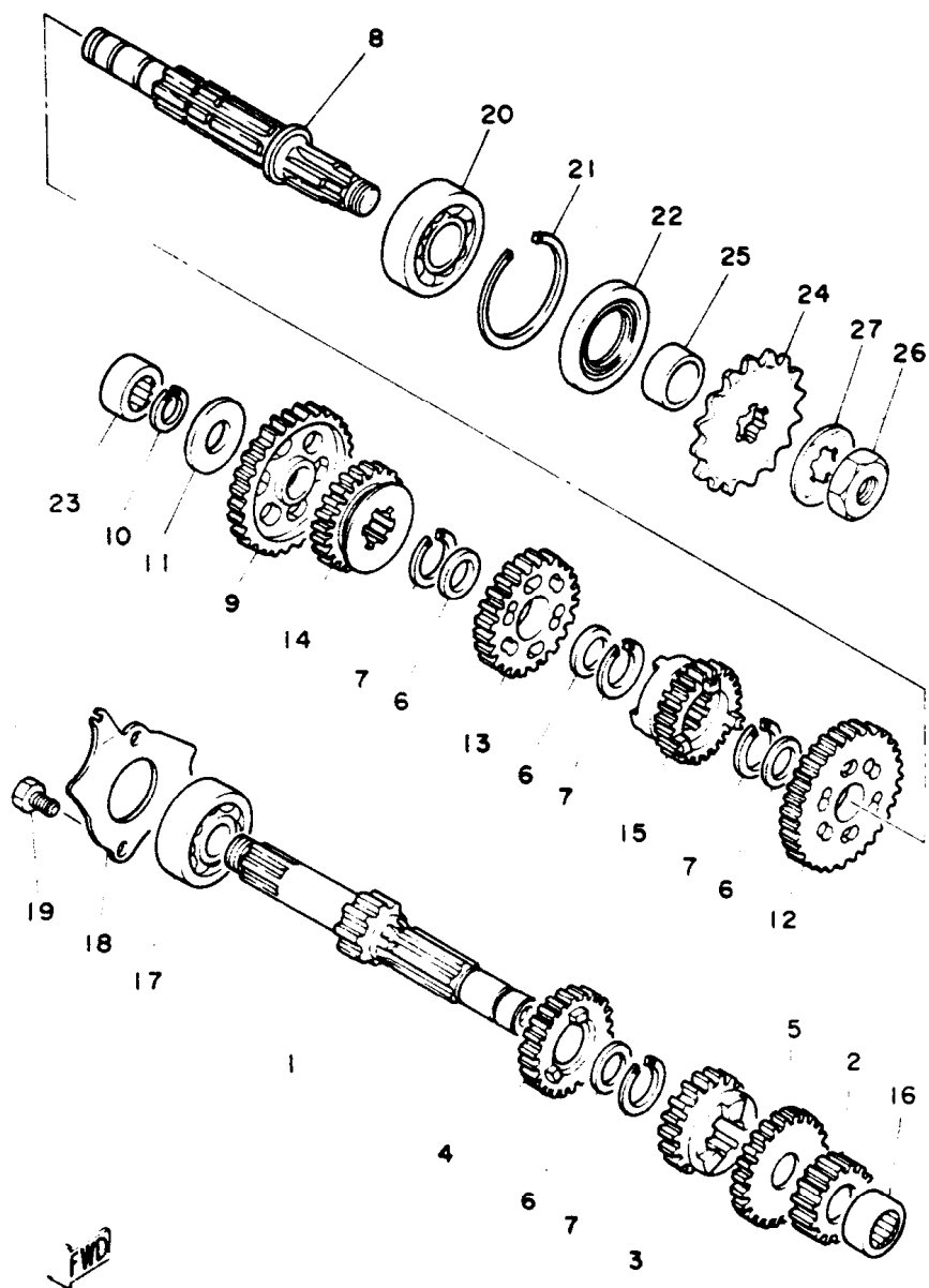
FIG. 11 – TRANSMISSÃO
