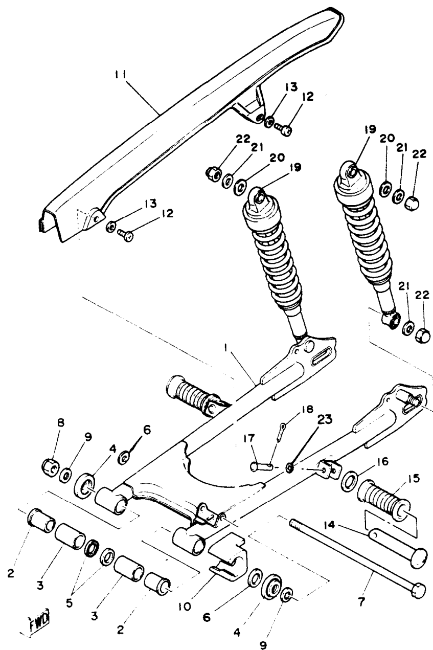
FIG. 19 – GARFO TRASEIRO
