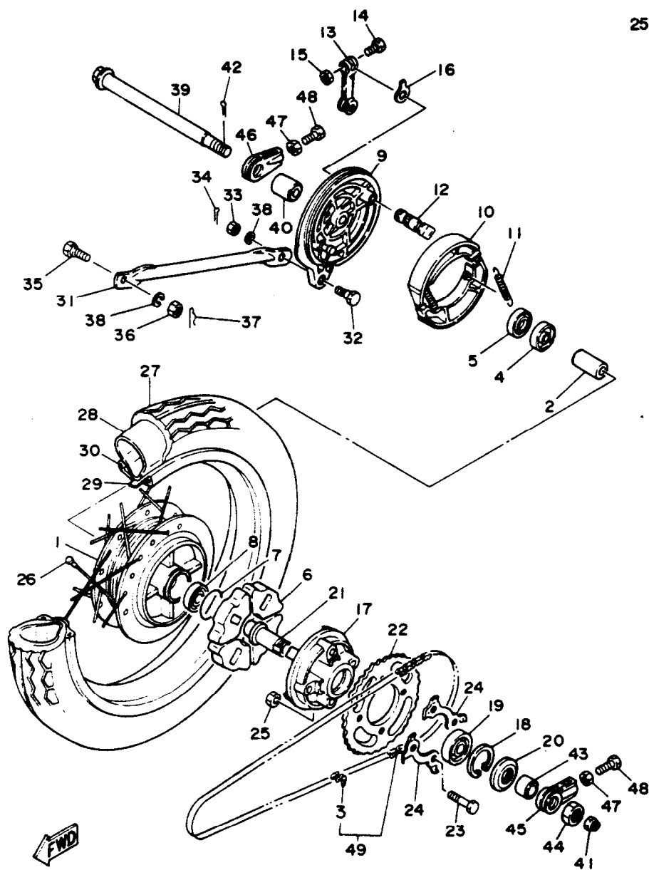
FIG. 25 - RODA TRASEIRA
