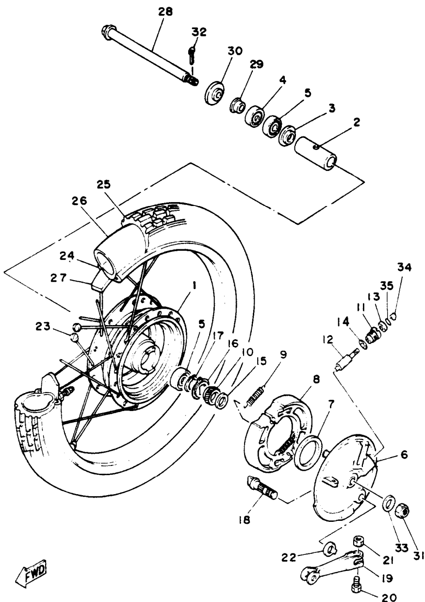
FIG. 24 – RODA DIANTEIRA
