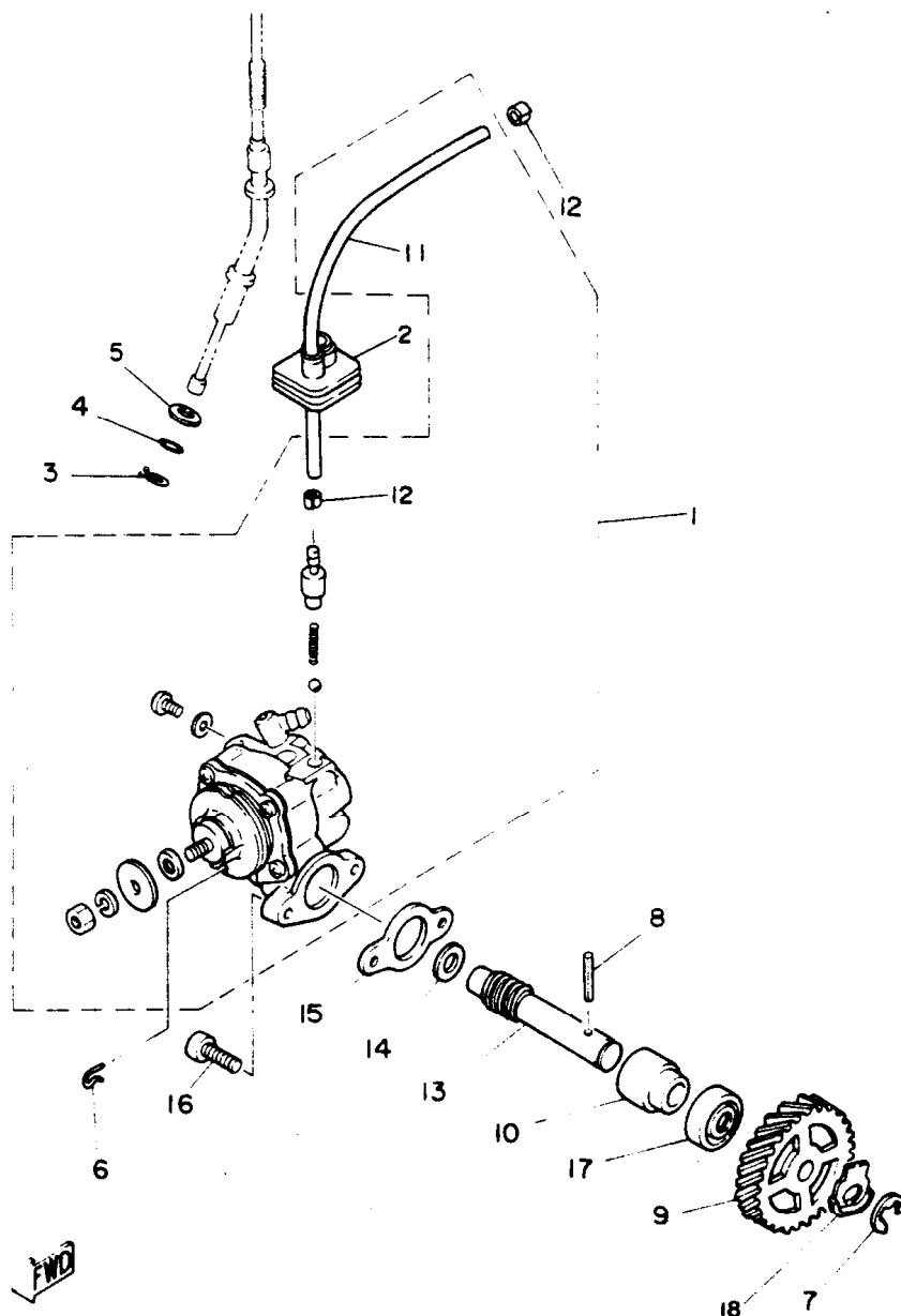
FIG. 3 – BOMBA DE ÓLEO
