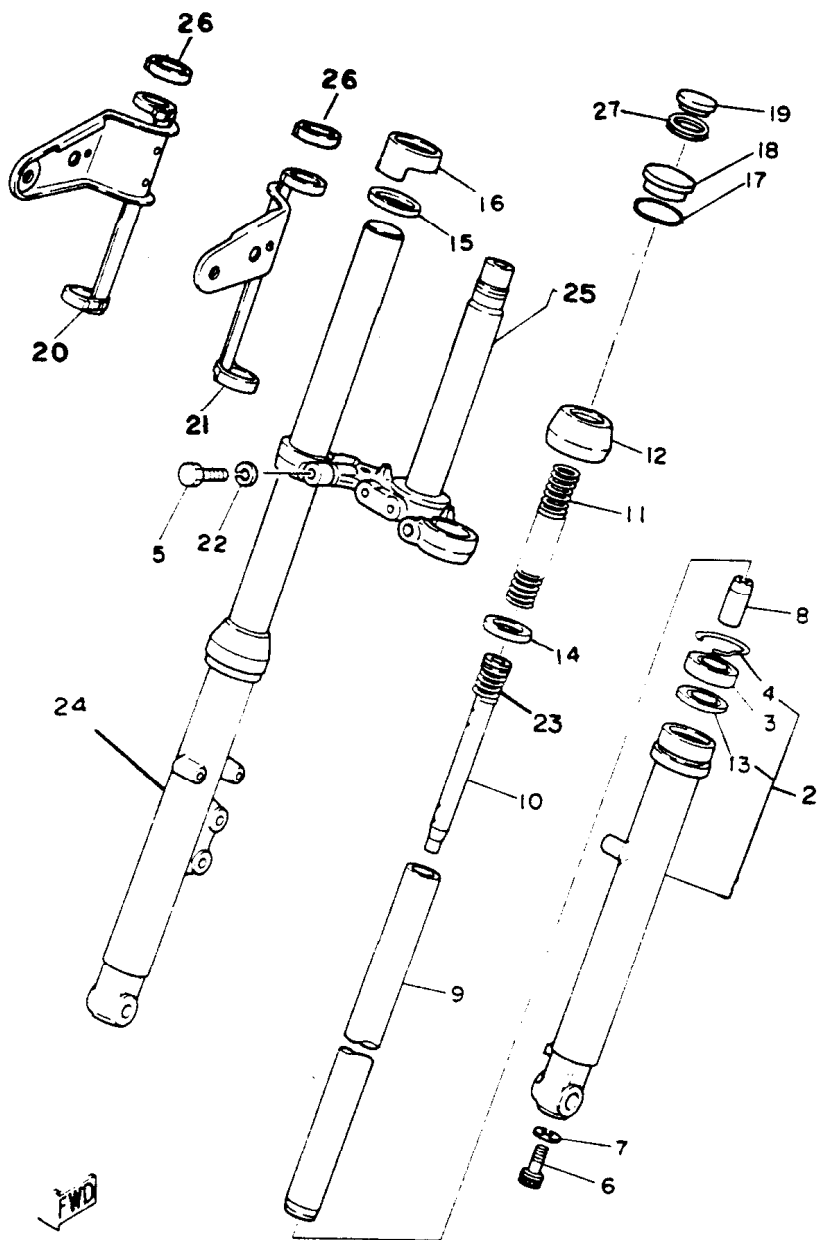
FIG. 21 – GARFO TELESCÓPICO
