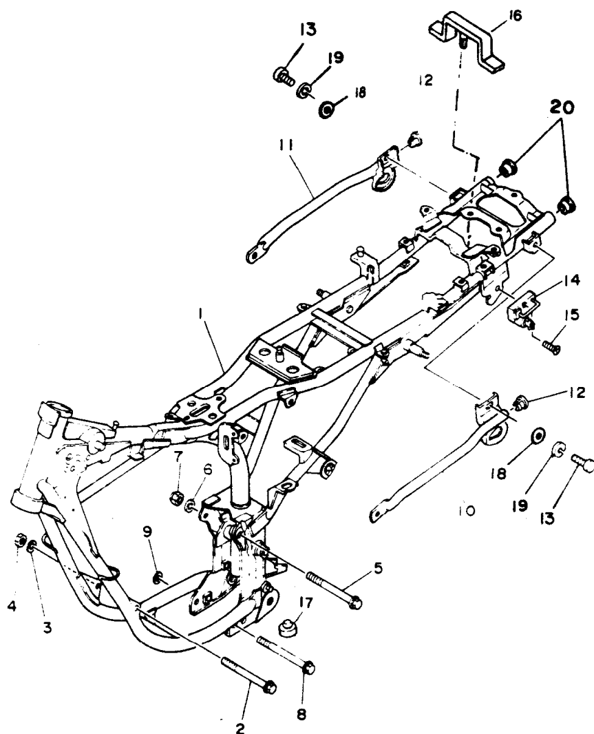
FIG. 15 – CHASSI
