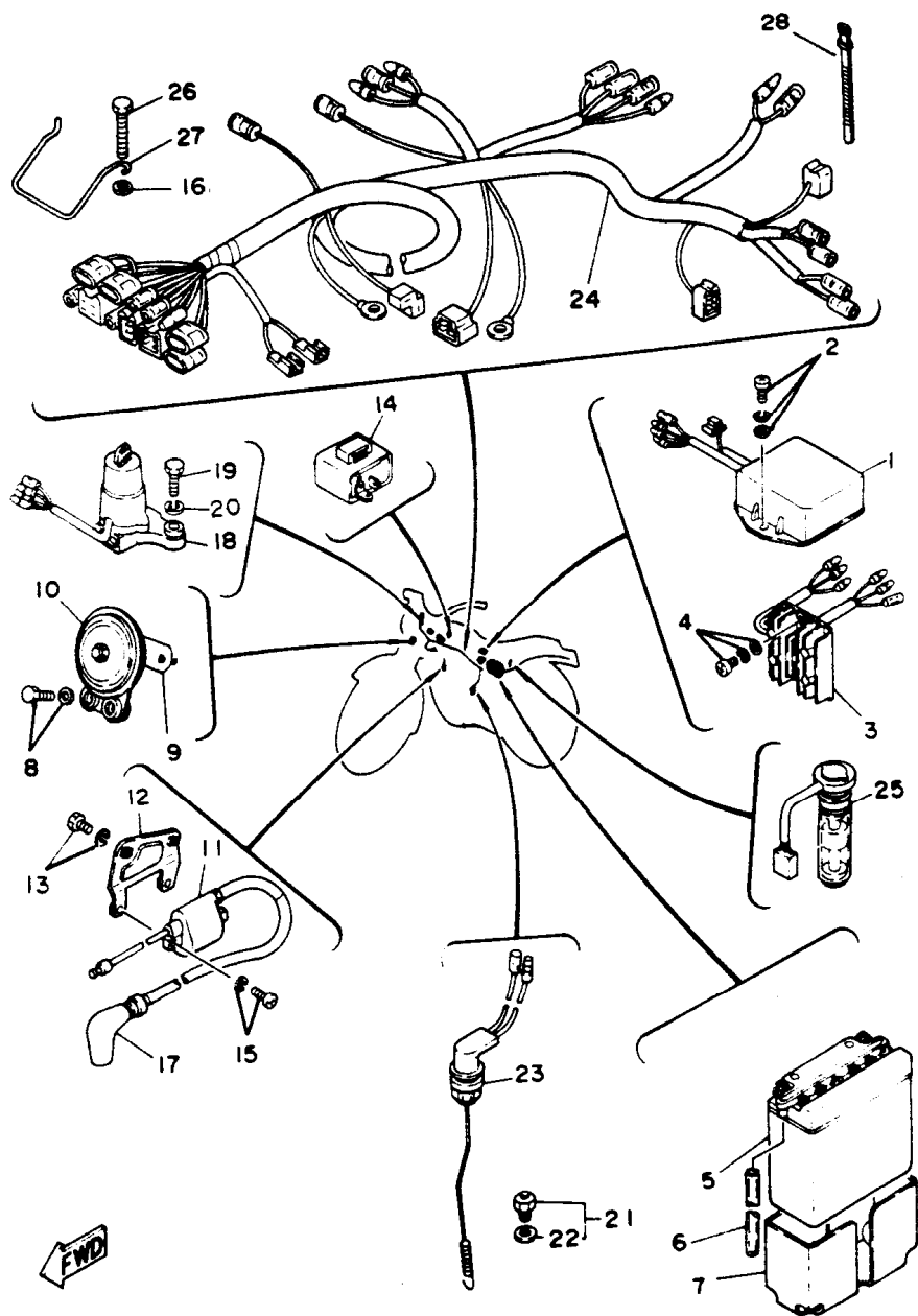
FIG. 33 – SISTEMA ELÉTRICO
