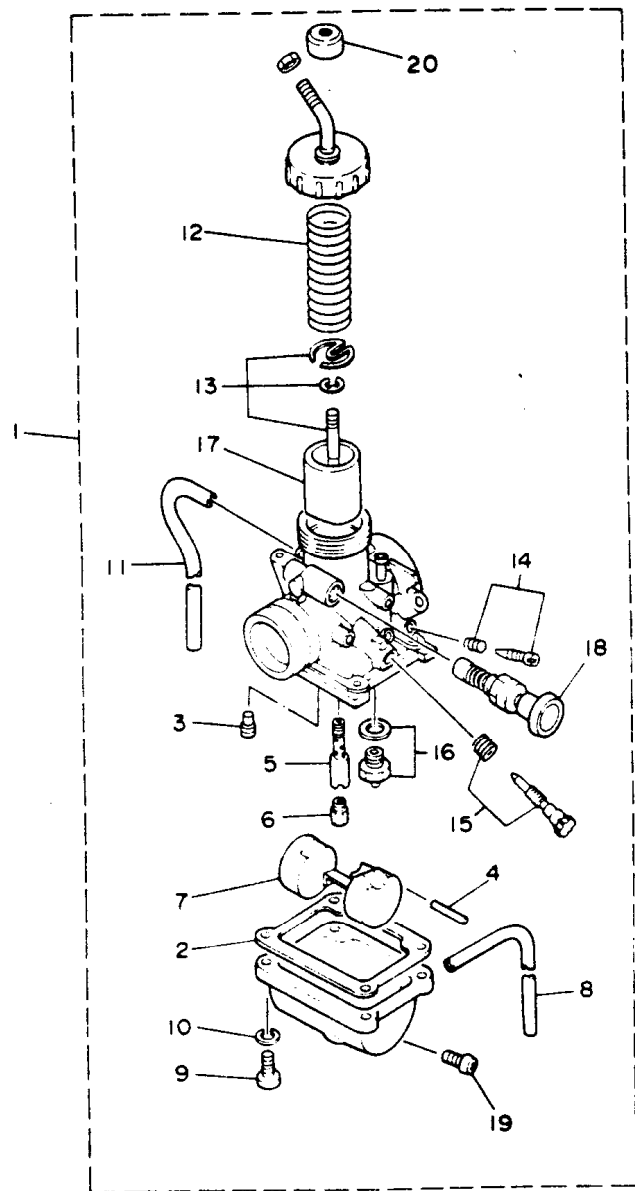
FIG. 5 – CARBURADOR
