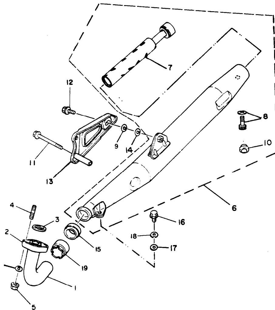
FIG. 6 – ESCAPAMENTO
