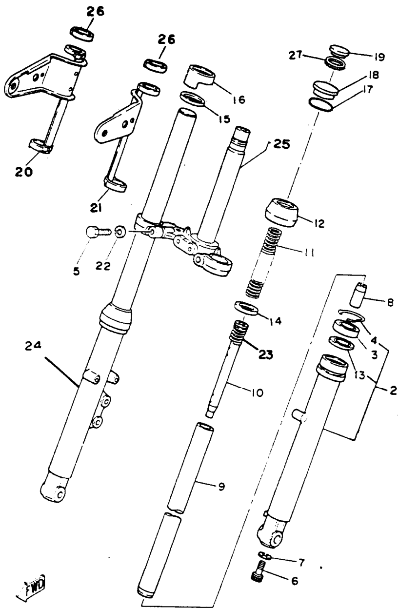
FIG. 21 – GARFO TELESCÓPICO
