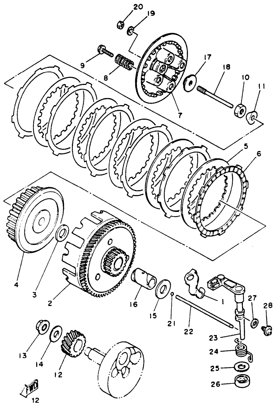
FIG. 10 – FRICÇÃO
