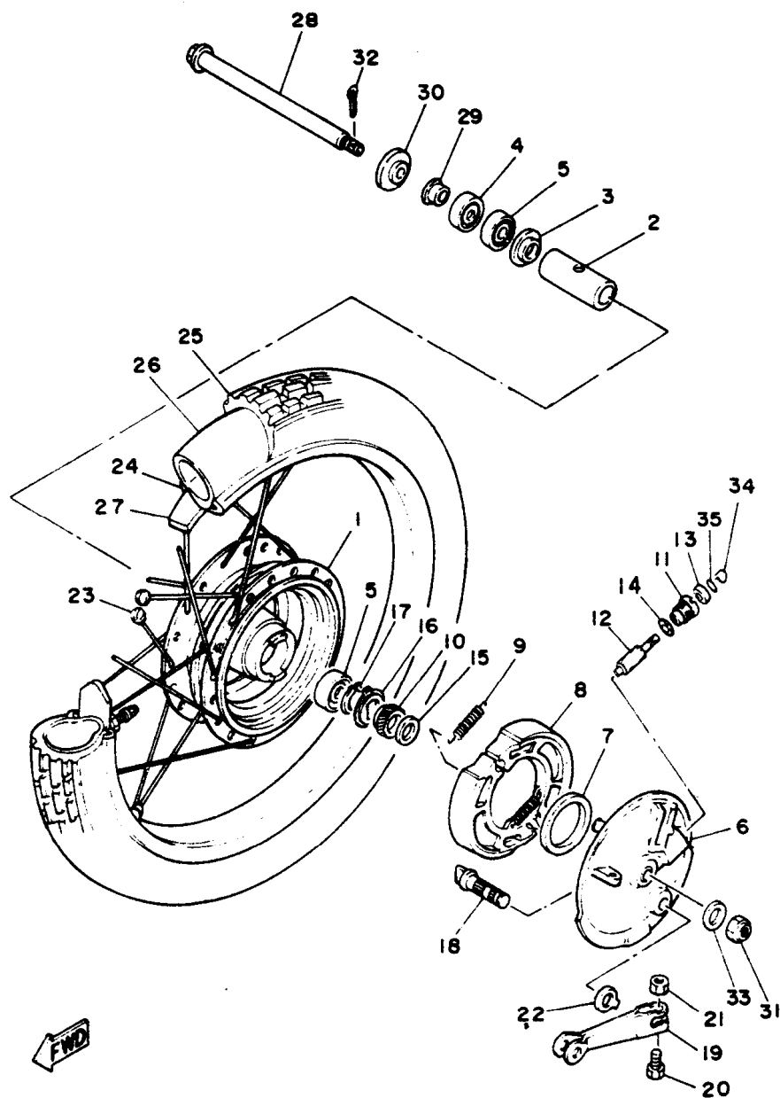
FIG. 24 – RODA DIANTEIRA
