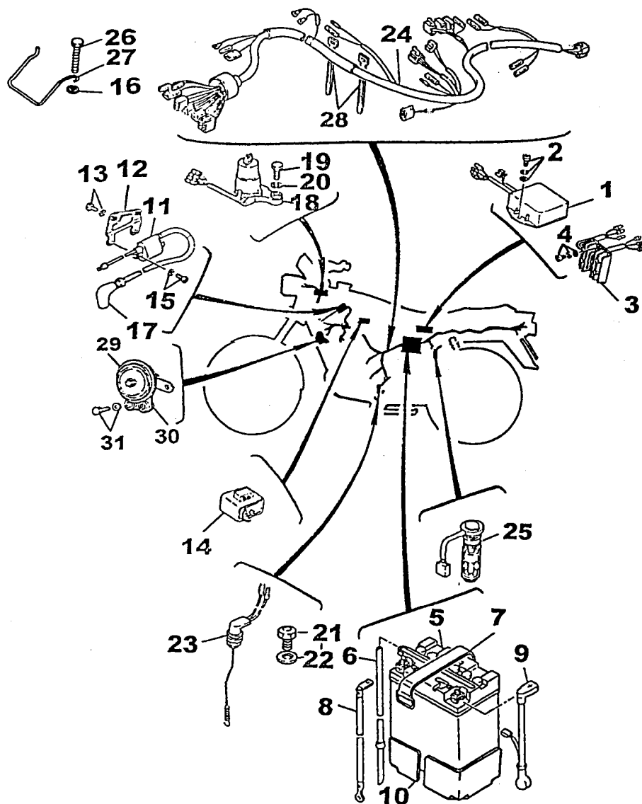
FIG. 33 - SISTEMA ELÉTRICO
