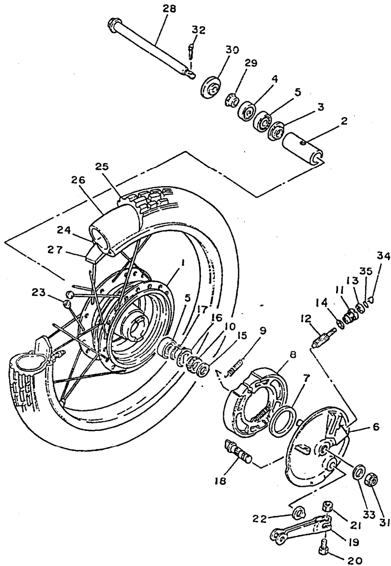
FIG. 24 - RODA DIANTEIRA
