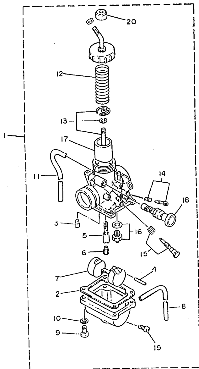
FIG. 5 - CARBURADOR
