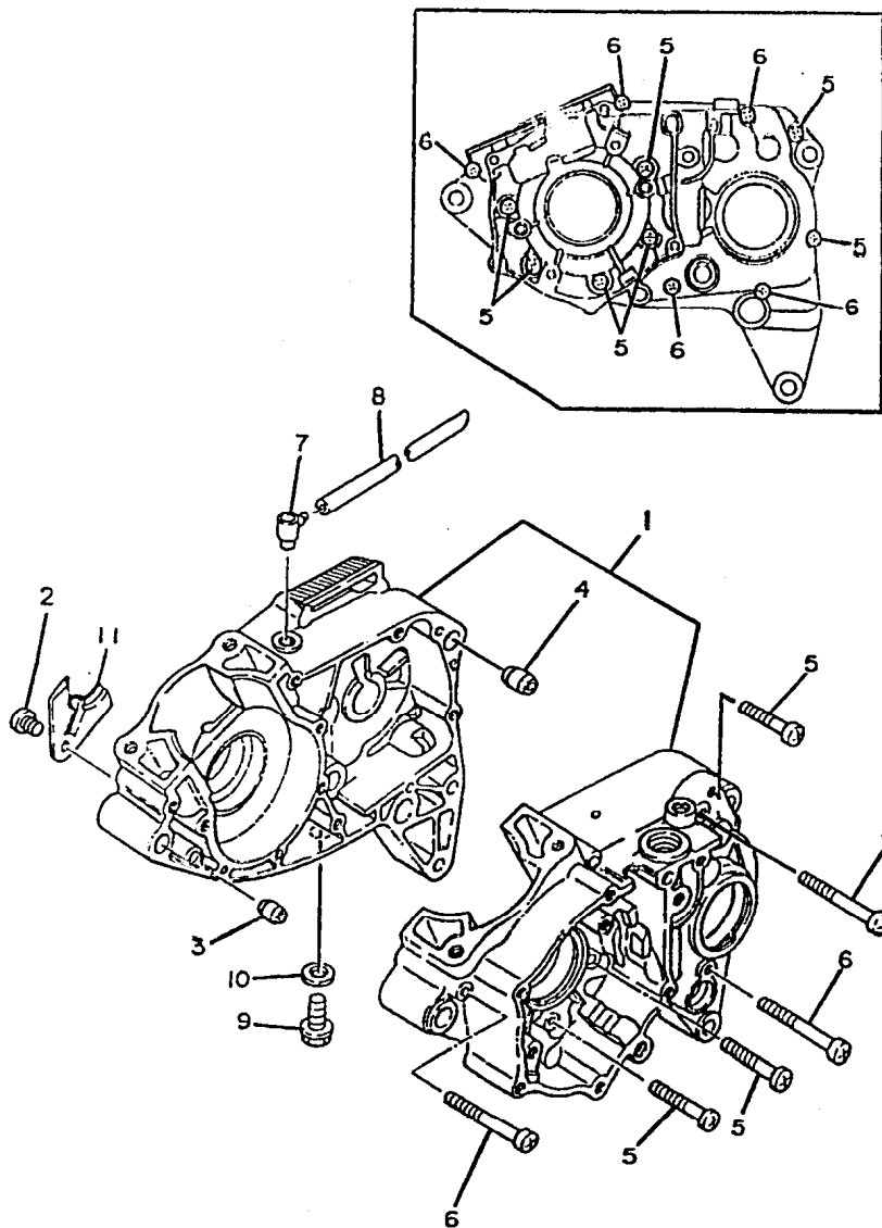
FIG. 07 - CARÇA DO MOTOR
