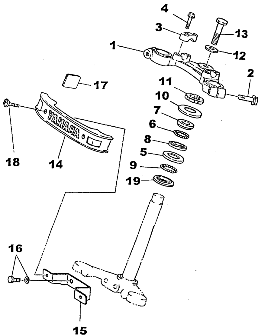
FIG. 20 - MESA DO GUIDÃO
