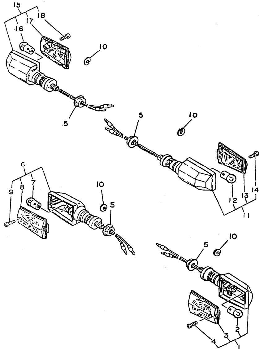
FIG. 29 - SINALIZADORES (PISCA-PISCA)
