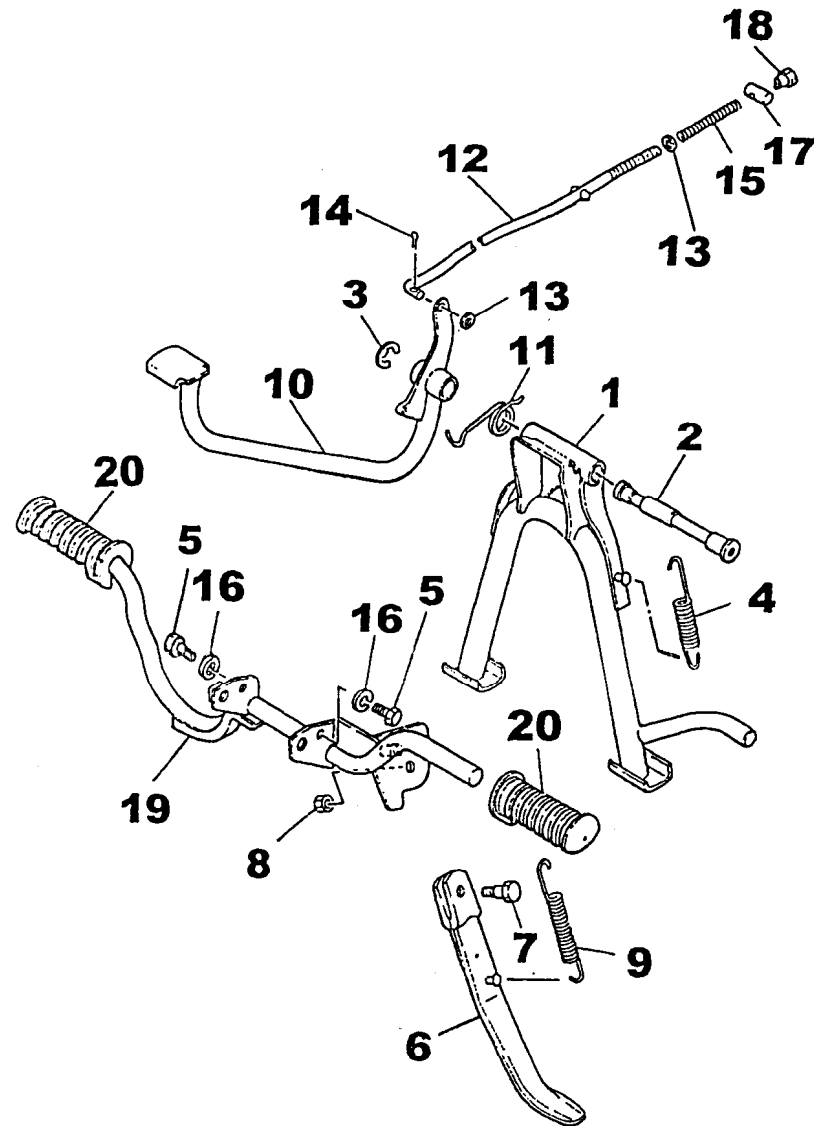
FIG. 27 - CAVALETES ESTRIBOS - PEDAL DE FREIO
