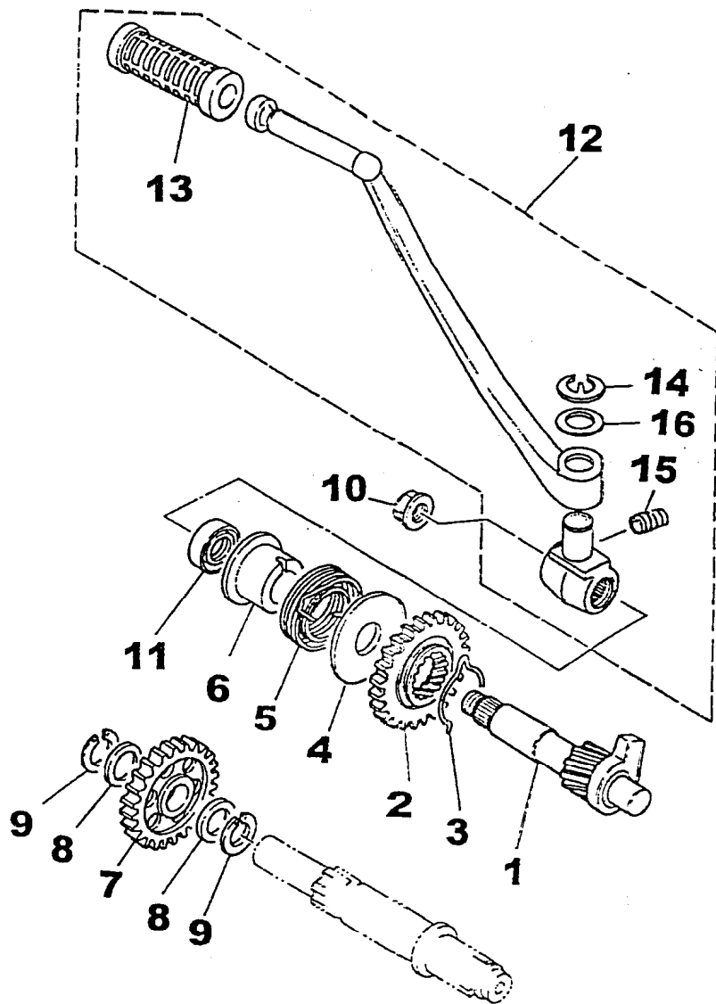
FIG. 9 - EIXO DO PEDAL DE PARTIDA
