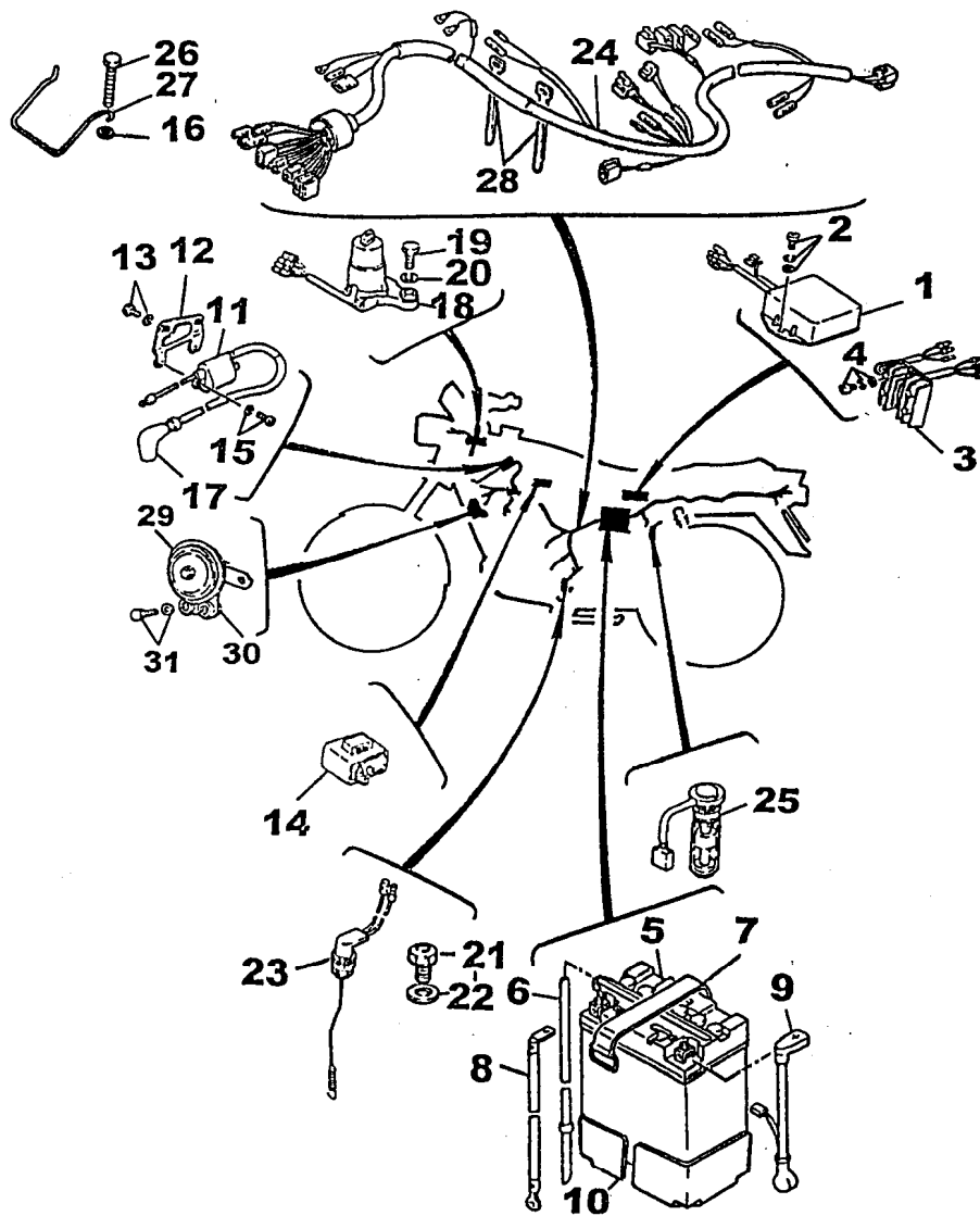
FIG. 33 - SISTEMA ELÉTRICO
