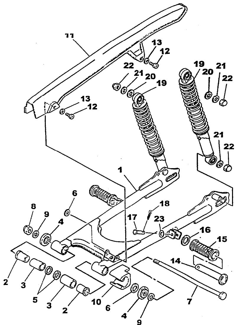
FIG. 19 - GARFO E AMORTECEDOR TRASEIRO
