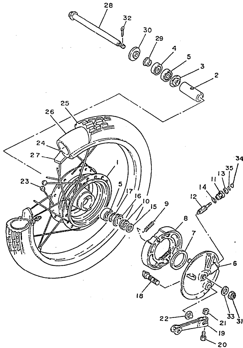
FIG. 24 - RODA DIANTEIRA
