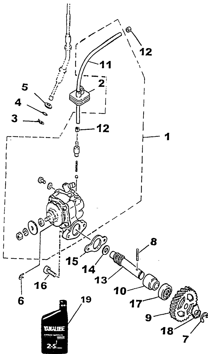
FIG. 3 - BOMBA DE ÓLEO
