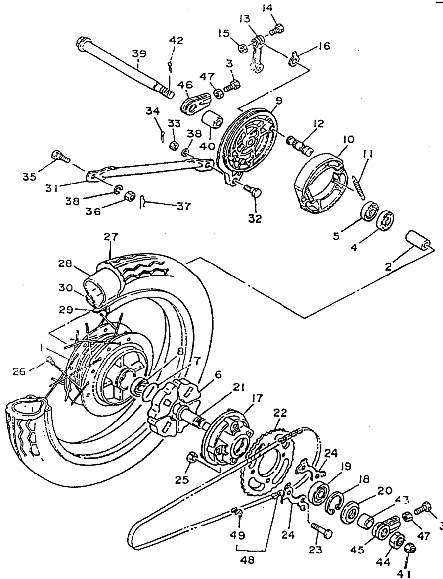
FIG. 25 - RODA TRASEIRA
