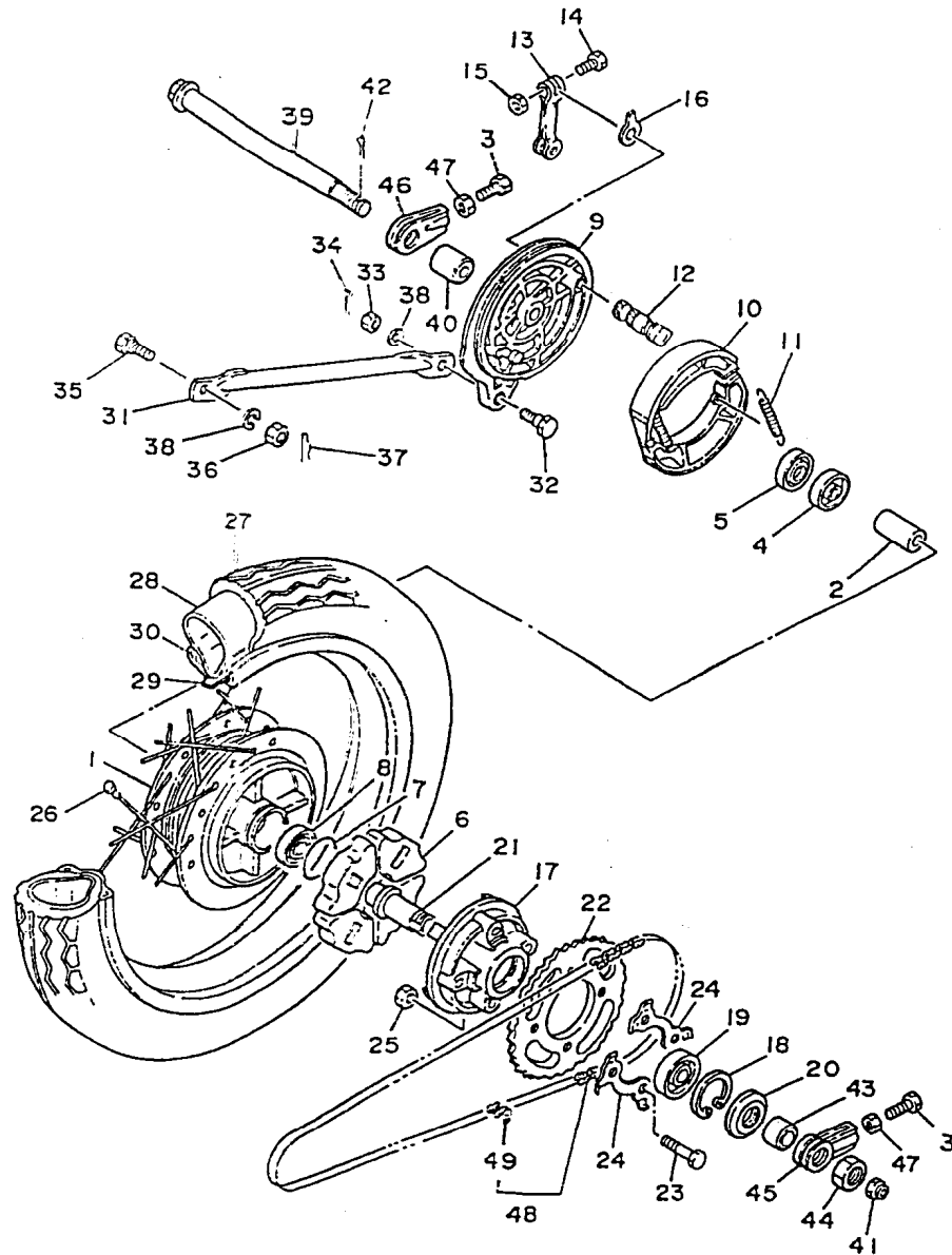
FIG. 25 - RODA TRASEIRA
