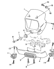
FIG.32 CARENAGEM P.42
