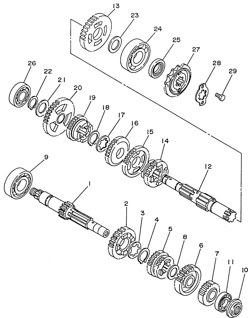
FIG. 14 - TRANSMISSÃO
