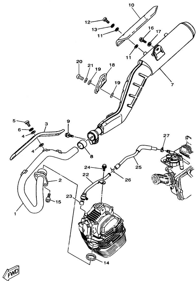
FIG. 09 - ESCAPAMENTO
