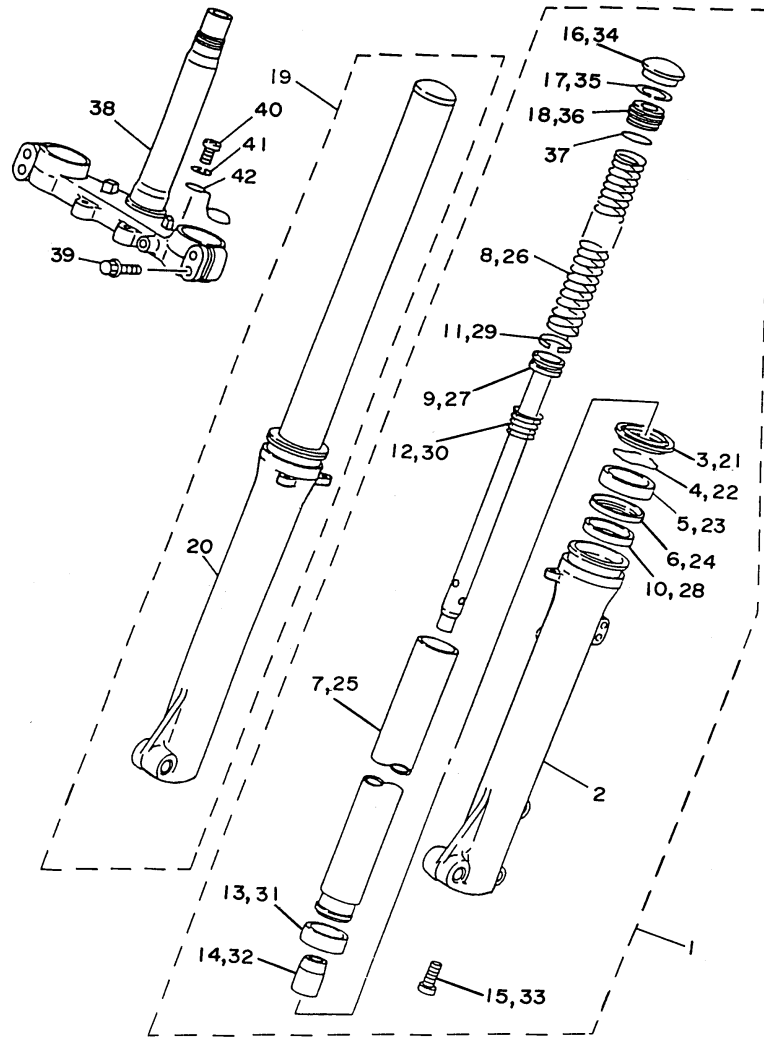
FIG. 23 - GARFO DIANTEIRO
