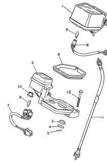
FIG.36 VELOCÍMETRO P.46
