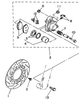
FIG.27 DISCO E PINÇA DE FREIO P.35
