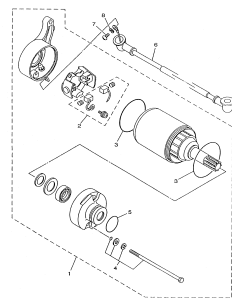
FIG.34 MOTOR DE PARTIDA P.44
