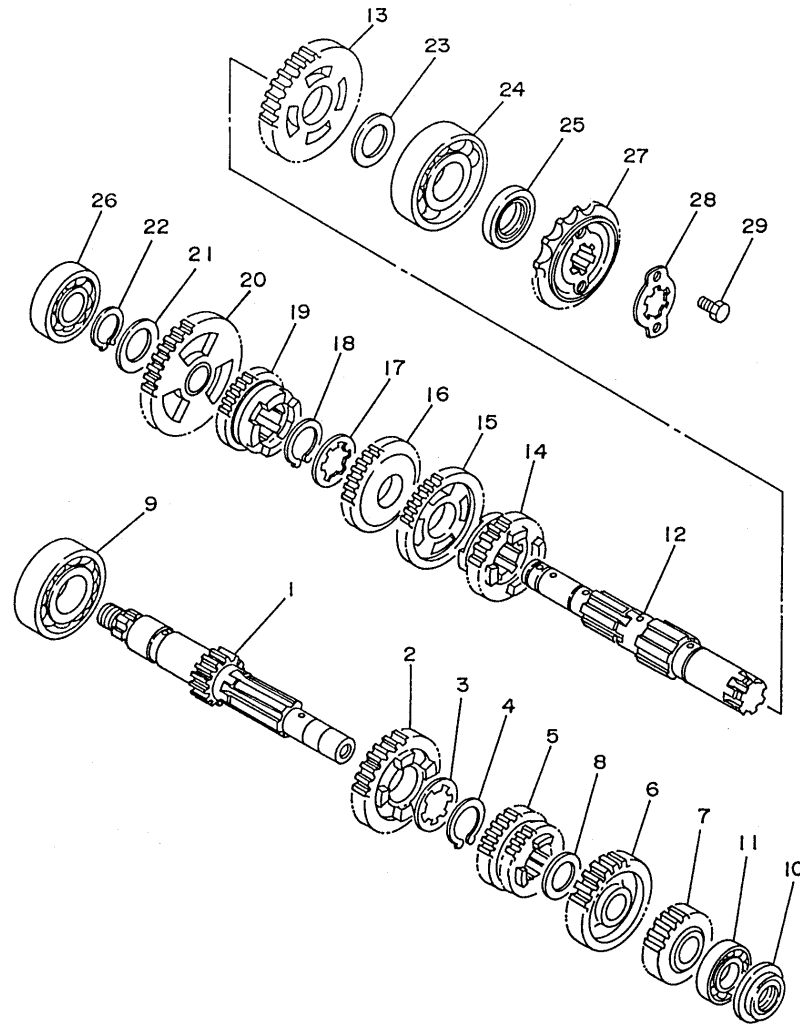
FIG. 14 - TRANSMISSÃO
