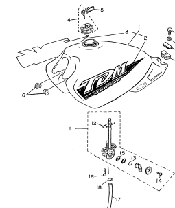
FIG.24 TANQUE DE COMBUSTÍVEL P.32
