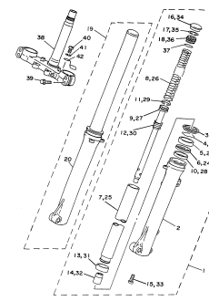
FIG.23 GARFO DIANTEIRO P.30 e P.31
