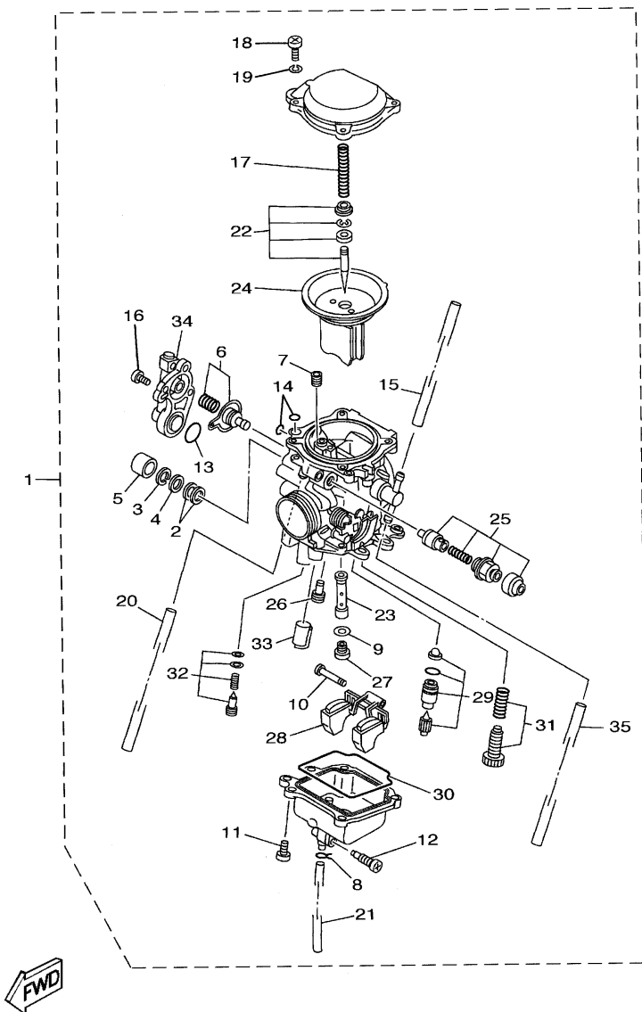
FIG. 08 - CARBURADOR
