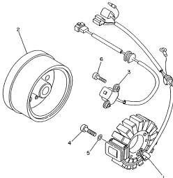
FIG.33 CONJUNTO MAGNETO P.43
