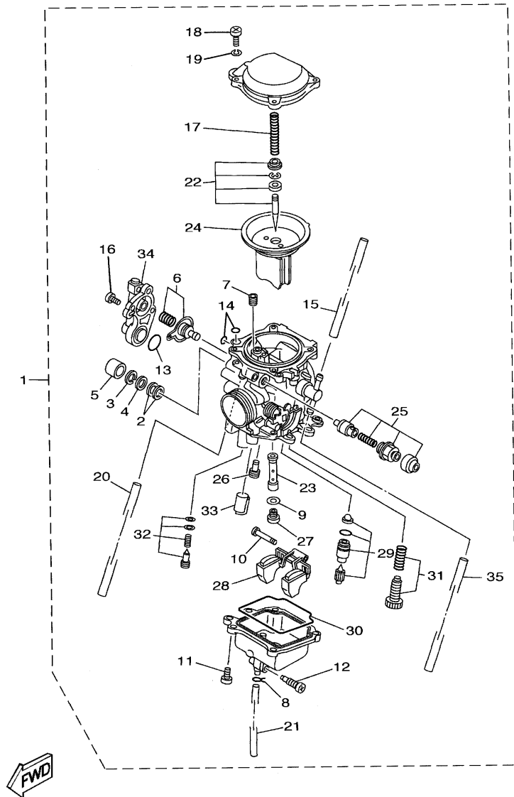
FIG. 08 - CARBURADOR
