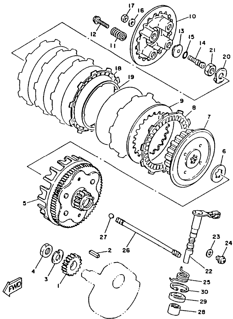
FIG. 12 - FRICÇÃO
