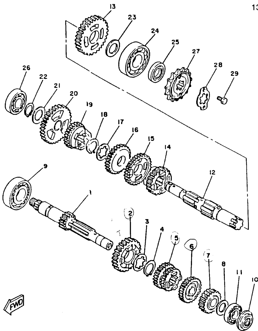
FIG. 13 - TRANSMISSÃO
