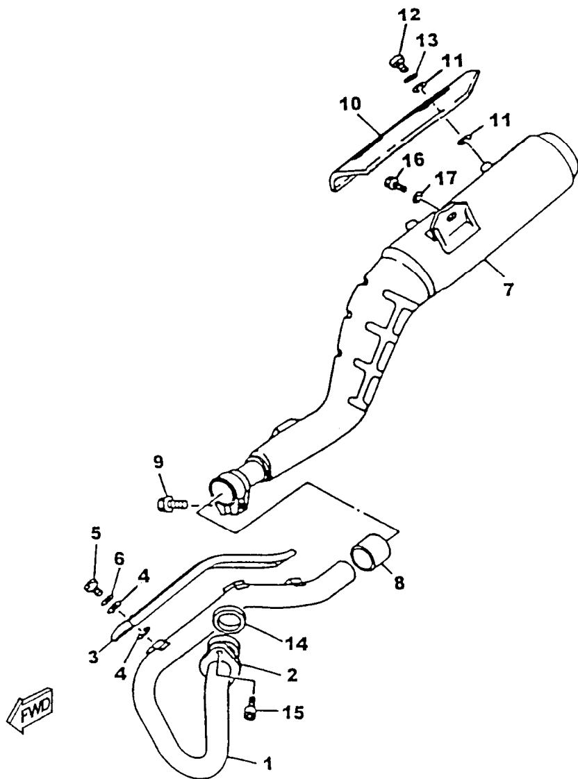
FIG. 08 - ESCAPAMENTO
