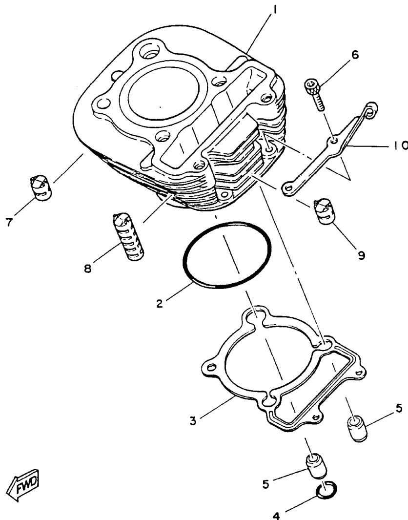
FIG. 02 - CILINDRO
