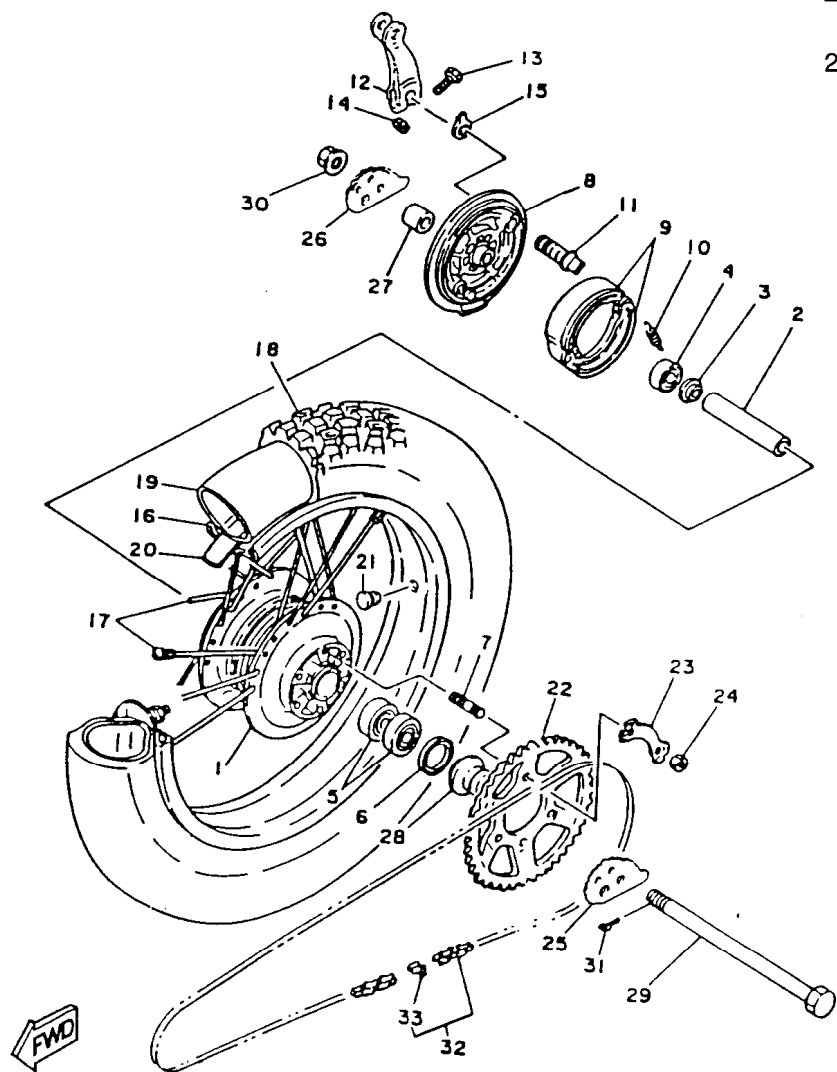
FIG. 24 - RODA TRASEIRA
