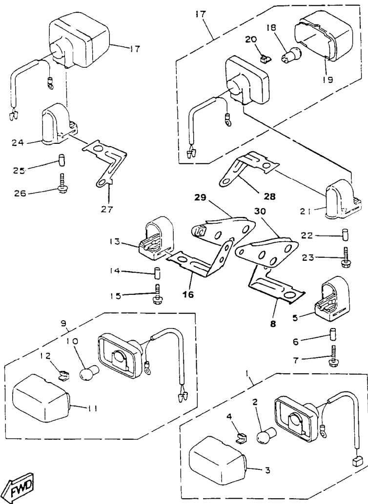
FIG. 37 - SINALIZADORES (PISCA-PISCA)
