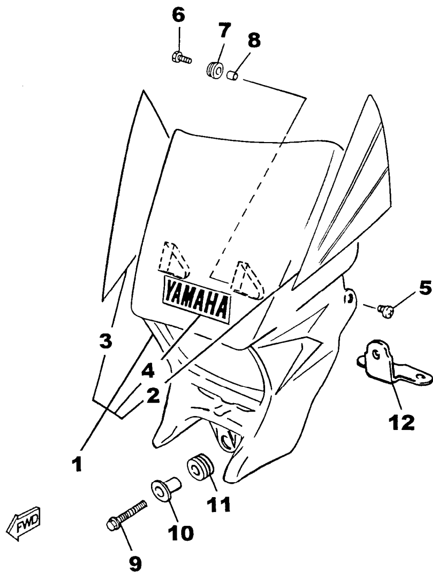
FIG. 28 - CARENAGEM
