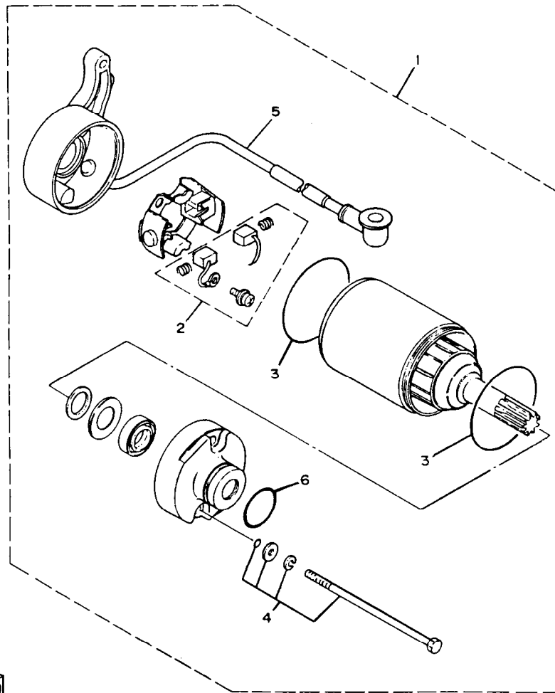
FIG. 39 - MOTOR DE PARTIDA
