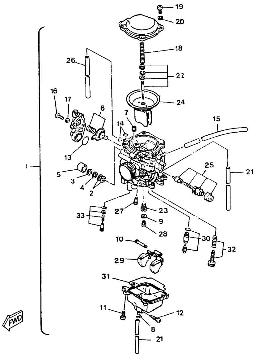
FIG. 16 - CARBURADOR
