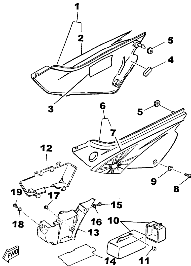
FIG. 29 - TAMPAS LATERAIS
