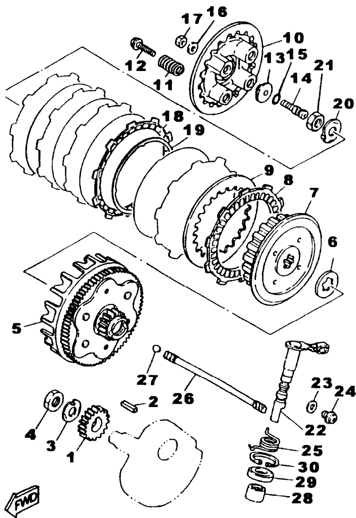
FIG. 12 - FRICÇÃO
