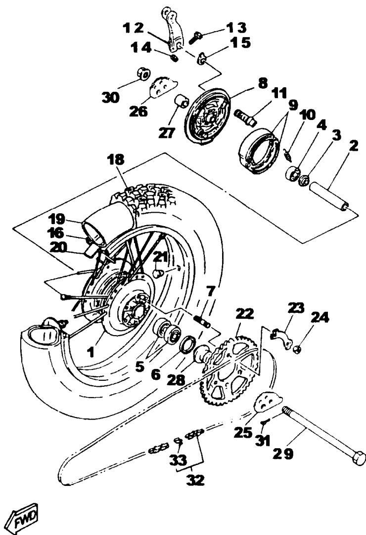
FIG. 24 - RODA TRASEIRA
