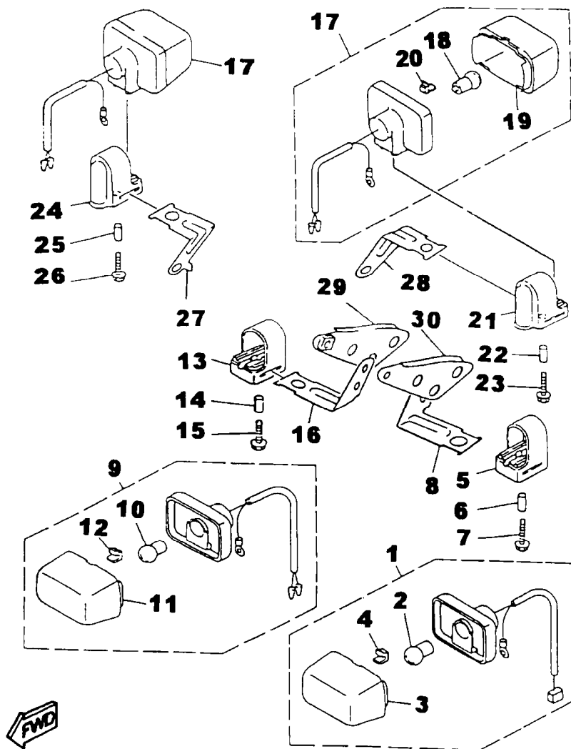
FIG. 37 - SINALIZADORES (PISCA-PISCA)
