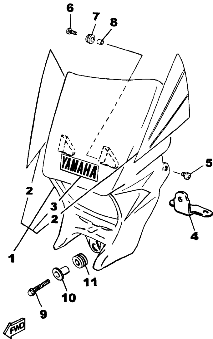
FIG. 28 - CARENAGEM
