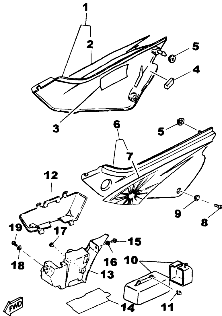
FIG. 29 - TAMPAS LATERAIS
