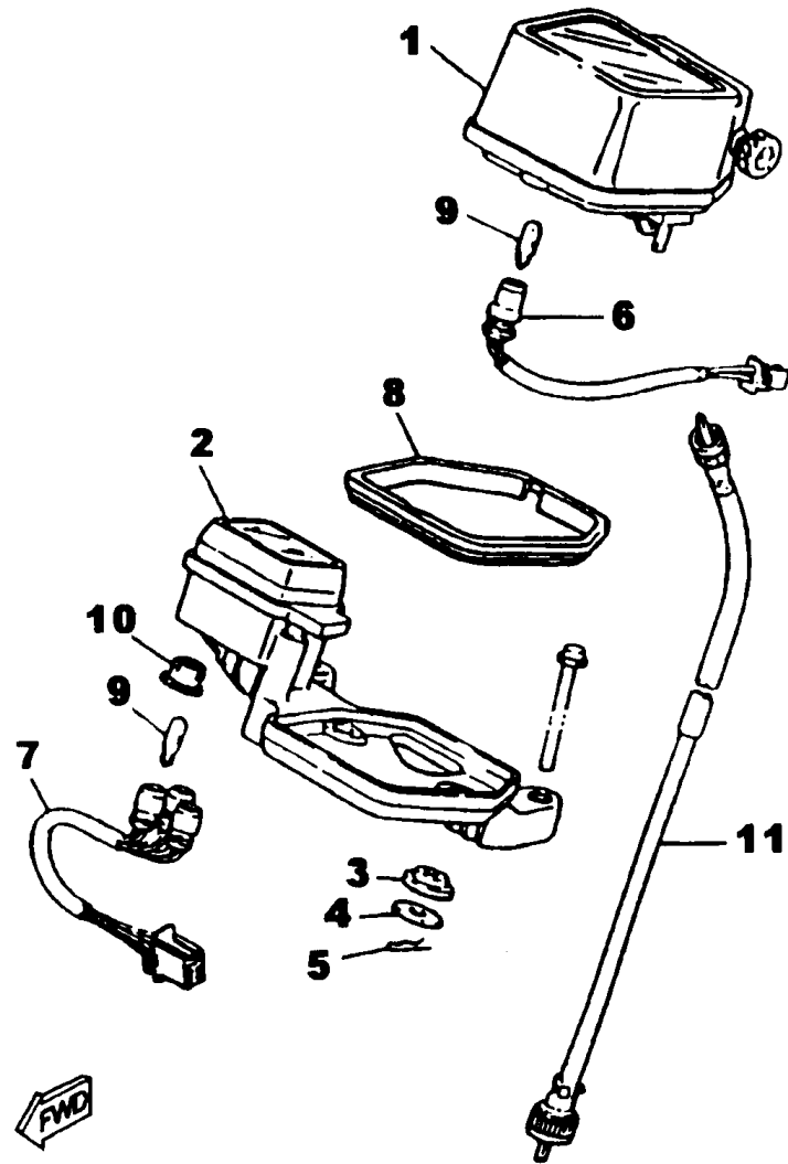
FIG. 38 - VELOCÍMETRO
