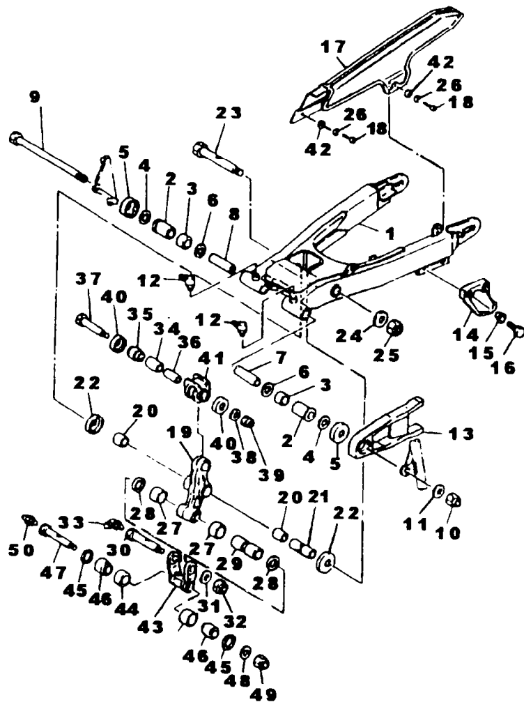
FIG. 19 - GARFO TRASEIRO
