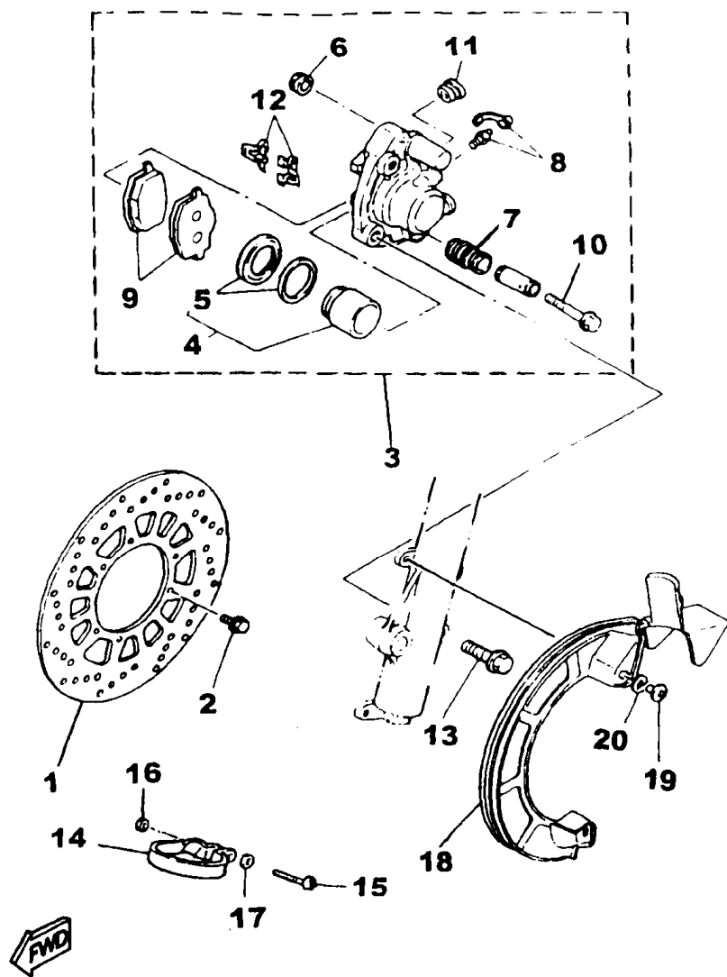
FIG. 23 - DISCO E PINÇA DO FREIO
