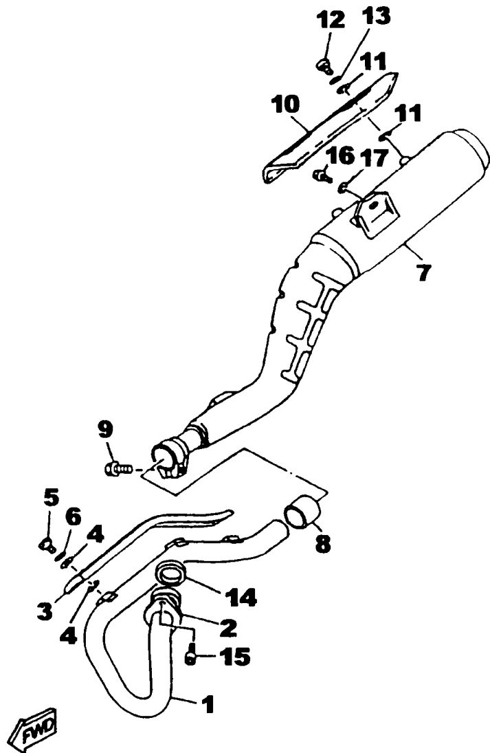
FIG. 08 - ESCAPAMENTO
