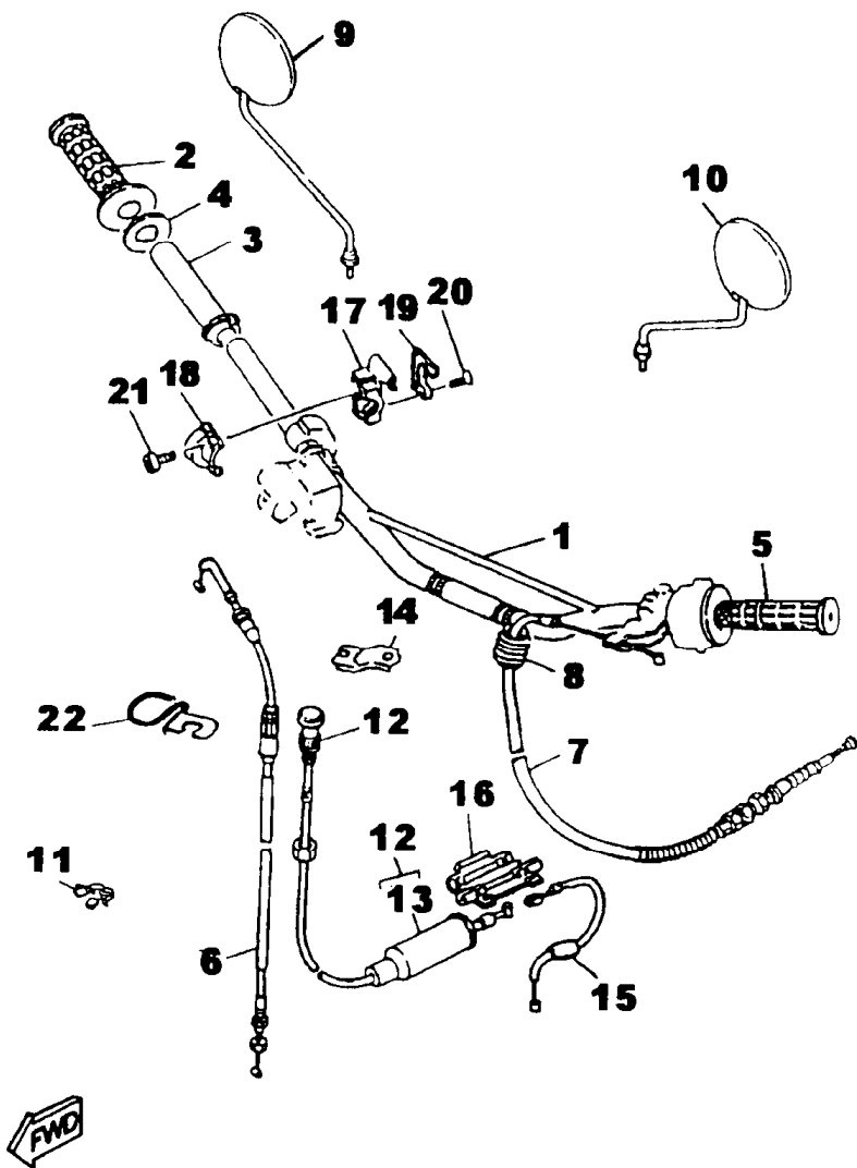
FIG. 31 - GUIDÃO E CABOS
