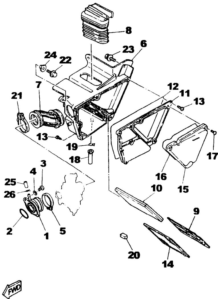
FIG. 07 - FILTRO DE AR
