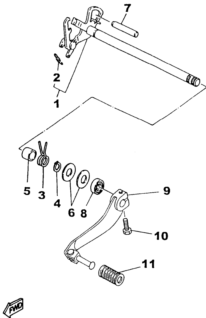
FIG. 15 - EIXO E PEDAL DE CÂMBIO
