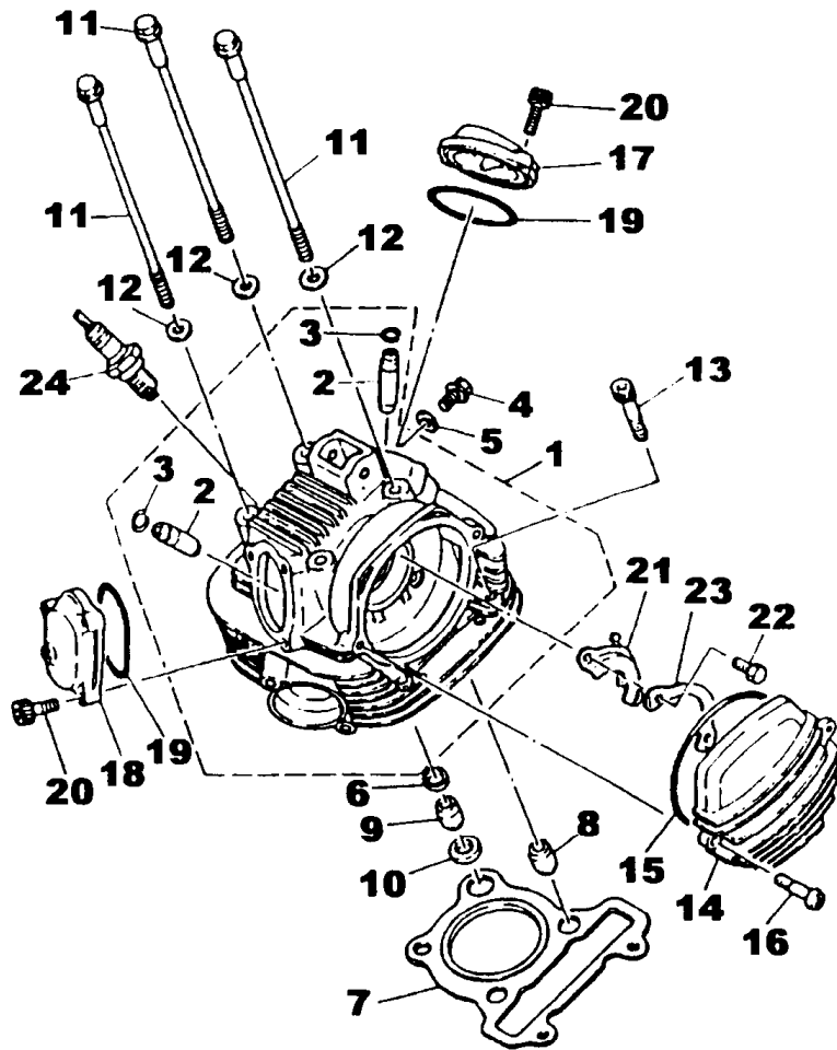
FIG. 01 - CABEÇOTE DO CILINDRO
