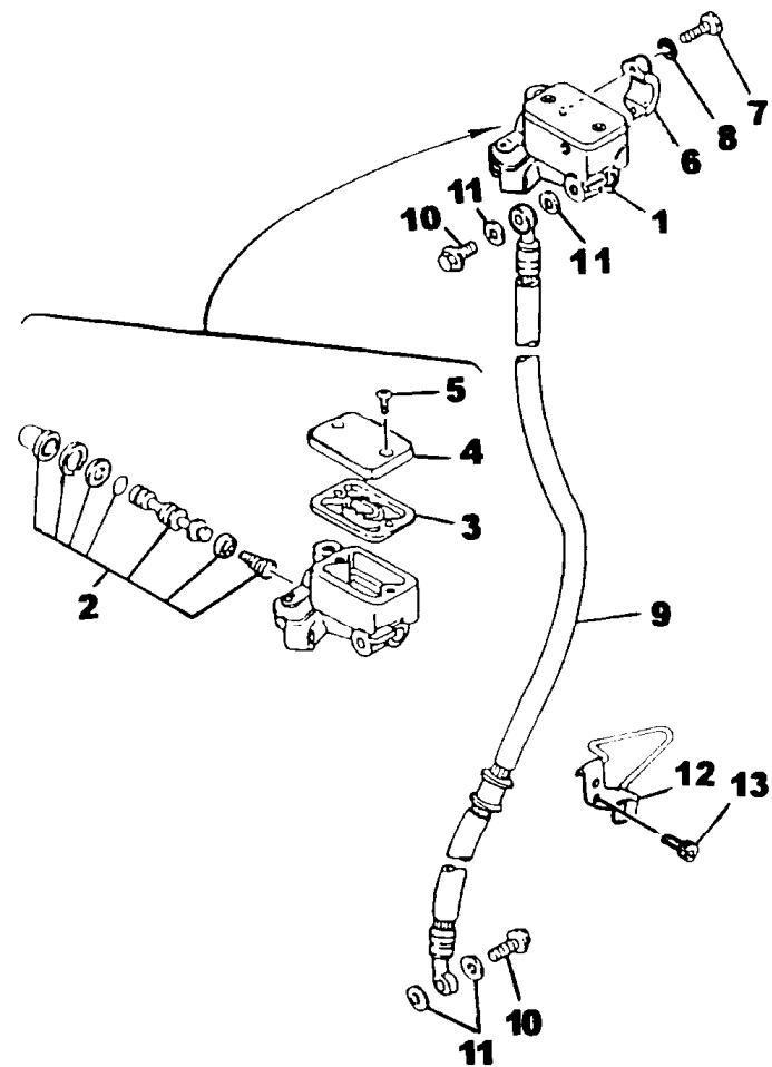
FIG. 33 - CILINDRO MESTRE
