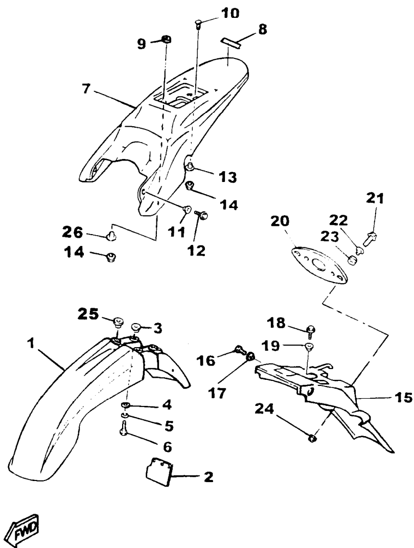
FIG. 18 - PÁRA-LAMAS DIANTEIRO E TRASEIRO
