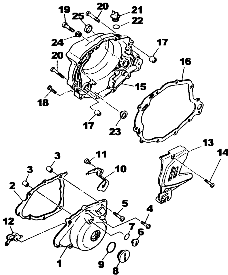
FIG. 10 - TAMPA DA CARÇAÇA
