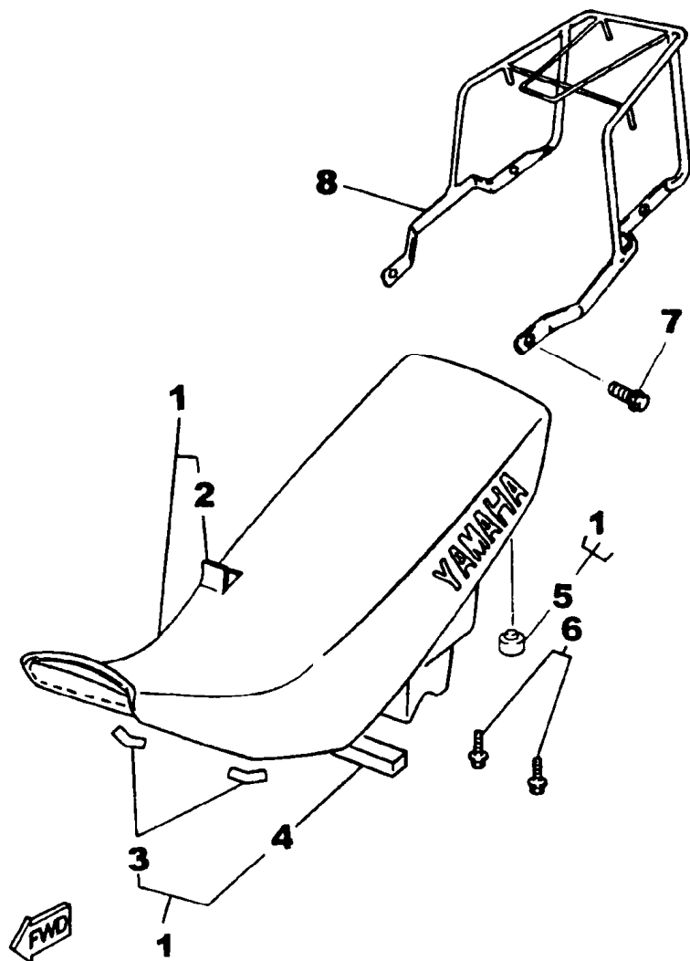
FIG. 26 - ASSENTO
