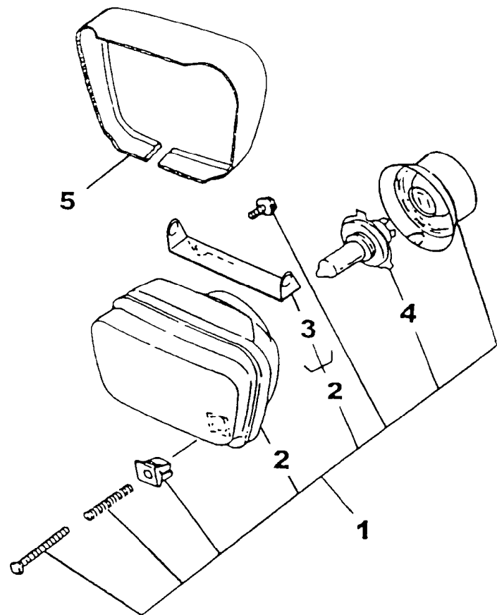
FIG. 32 - FAROL DIANTEIRO
