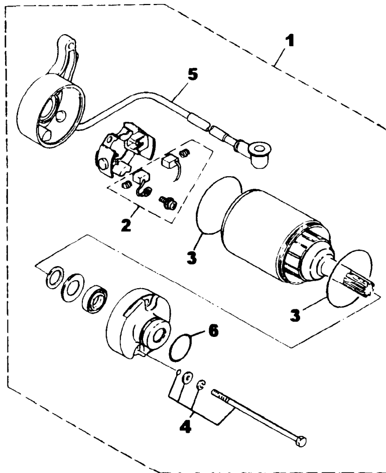
FIG. 39 - MOTOR DE PARTIDA
