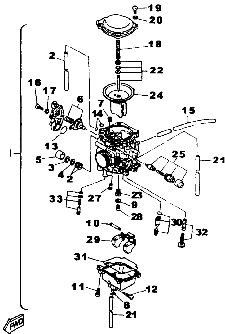
FIG. 16 - CARBURADOR
