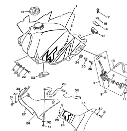
FIG.24 TANQUE DE COMBUSTÍVEL P.43 e P.44
