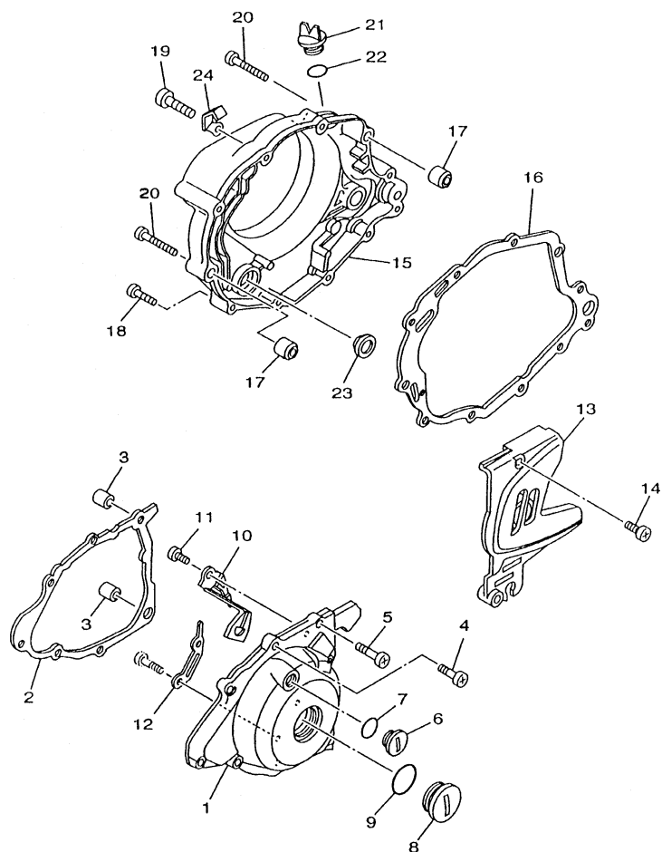
FIG. 11 - TAMPA DA CARÇAÇA
