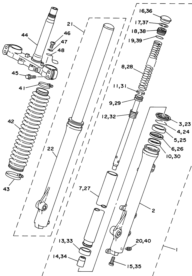
FIG. 23 - GARFO DIANTEIRO
