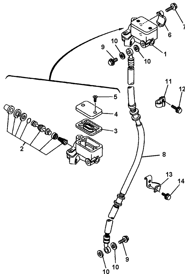
FIG. 30 - CILINDRO MESTRE
