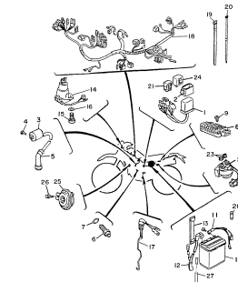
FIG.40 SISTEMA ELÉTRICO P.62
