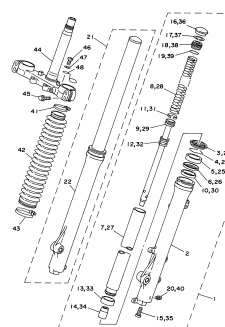
FIG.23 GARFO DIANTEIRO P.41 e P.42
