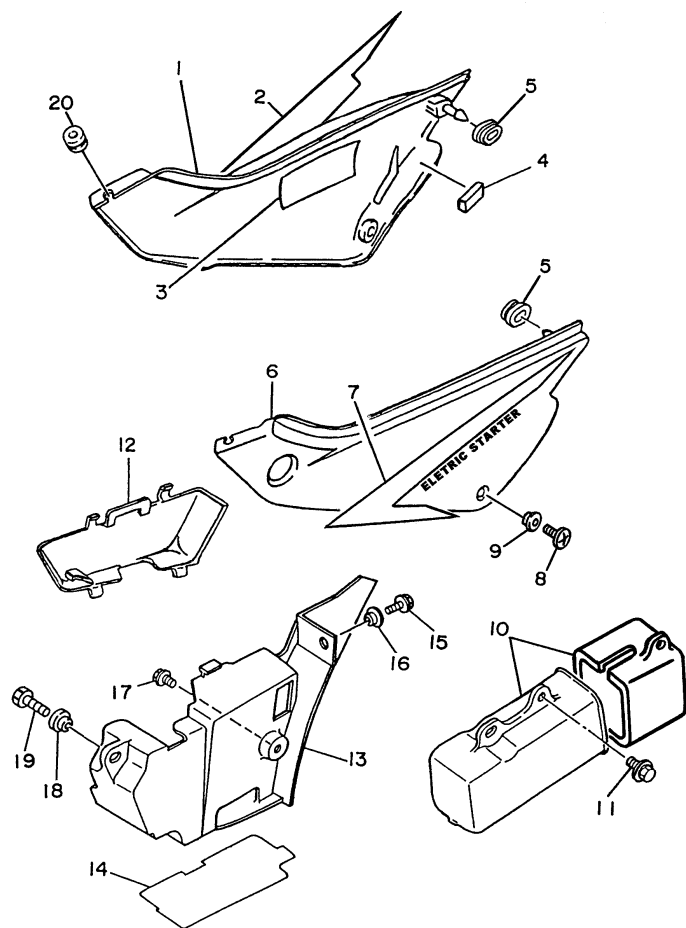
FIG. 19 - TAMPAS LATERAIS
