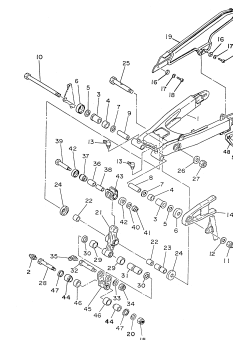
FIG.20 GARFO TRASEIRO P.37 e P.38
