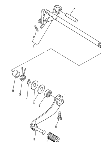
FIG.16 EIXO E PEDAL DE MUDANÇA P.32
