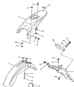
FIG.18 PÁRA-LAMAS DIANTEIRO E TRASEIRO P.35
