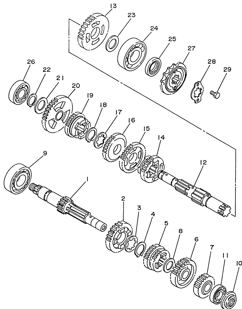
FIG. 14 - TRANSMISSÃO
