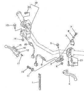
FIG.39 INTERRUPTOR DO GUIDÃO • MANETES P.61
