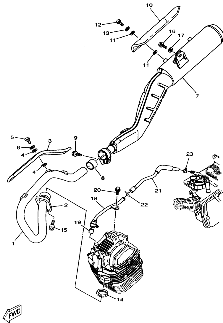
FIG. 09 - ESCAPAMENTO
