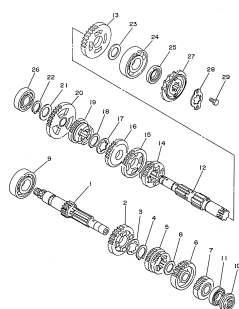
FIG.14 TRANSMISSÃO P.29 e P.30
