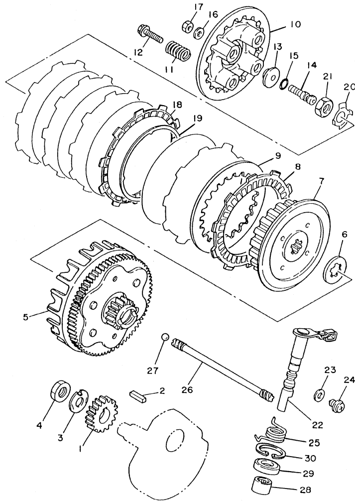
FIG. 13 - FRICÇÃO
