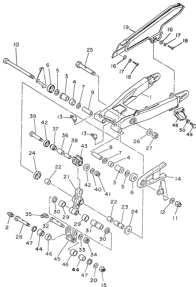
FIG. 20 - GARFO TRASEIRO
