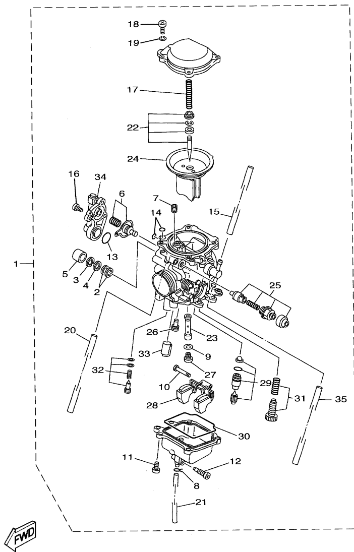
FIG. 08 - CARBURADOR
