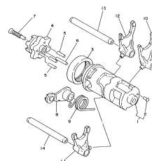
FIG.15 EIXO TRAMBULADOR P.31
