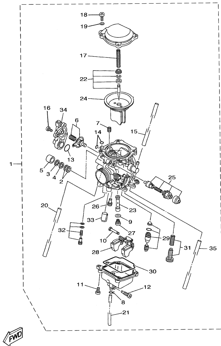
FIG. 08 - CARBURADOR
