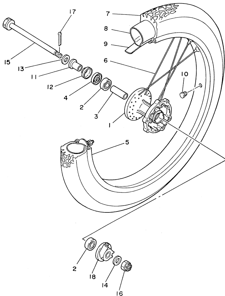
FIG. 26 - RODA DIANTEIRA
