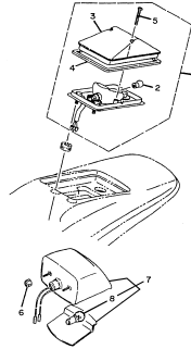
FIG.38 LANTERNA TRASEIRA P.60
