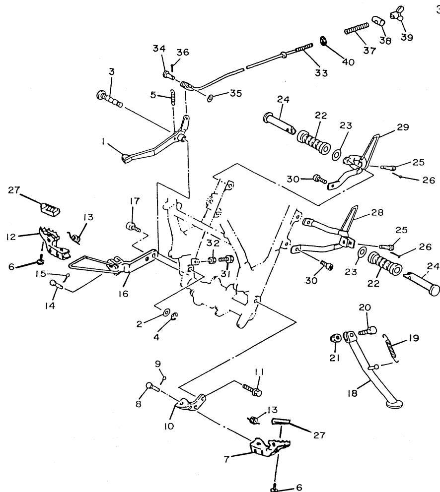
FIG. 31 - CAVALETE LATERAL - ESTRIBOS
