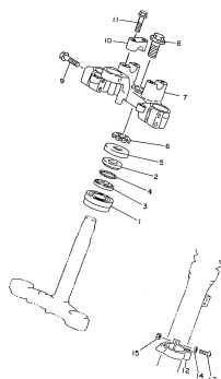
FIG.22 MESA DO GUIDÃO P.40
