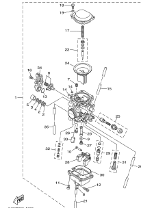
FIG. 8 CARBURADOR
