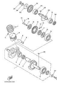
FIG. 3 VIRABREQUIM E PISTÃO
