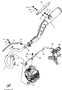
FIG. 9 ESCAPAMENTO
