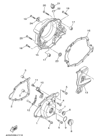
FIG. 11 TAMPA DA CARCAÇA
