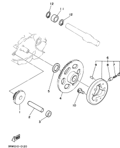
FIG. 12 EMBREAGEM DA PARTIDA
