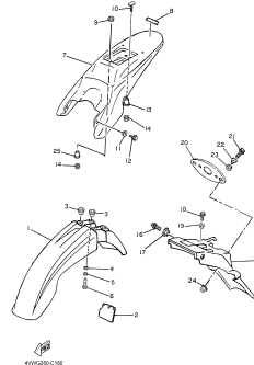
FIG.18 PÁRA-LAMA
