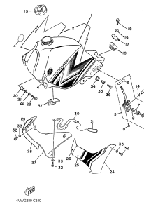
FIG. 24 TANQUE DE COMBUSTÍVEL
