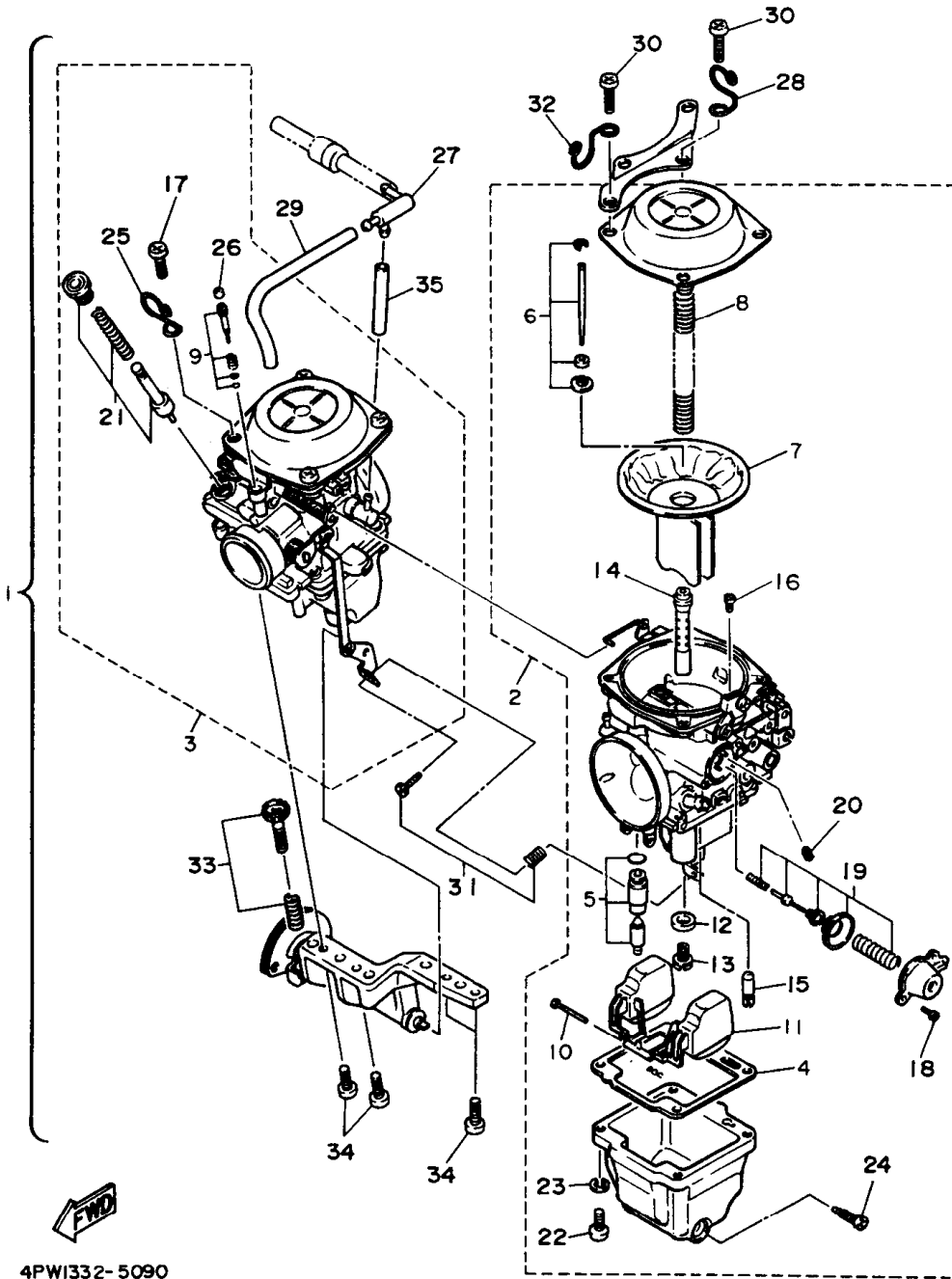
FIG. 9 CARBURETOR
