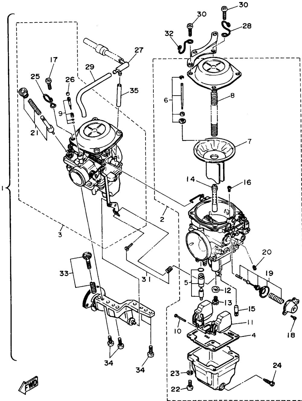
FIG. 9 CARBURETOR
